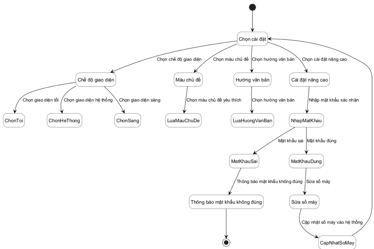
Hình 3.102: Sơ đồ trạng thái cho chức năng cài đặt ứng dụng student client
