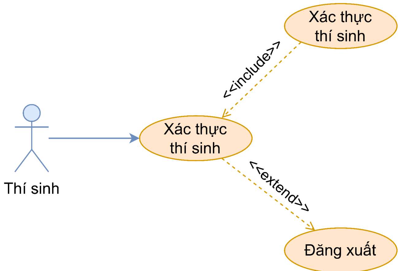
Hình 3.30: Phân rã use case Xác thực thí sinh
