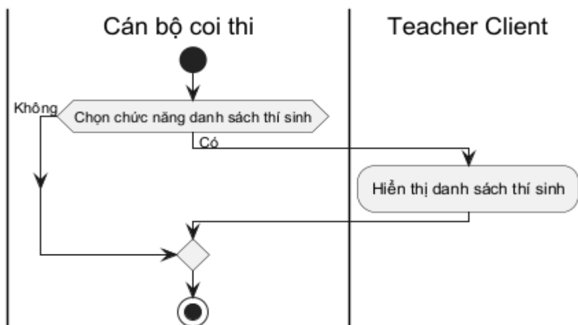
Hình 3.58: Sơ đồ hoạt động cho chức năng danh sách thí sinh
