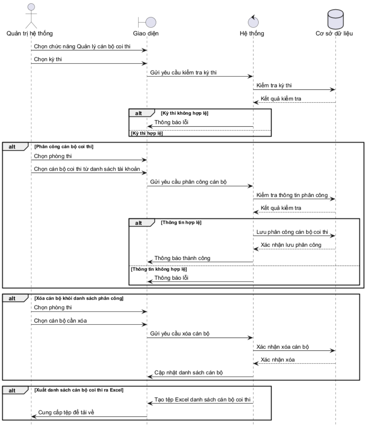
Hình 3.117: Sơ đồ tuần tự cho chức năng quản lý cán bộ coi thi
