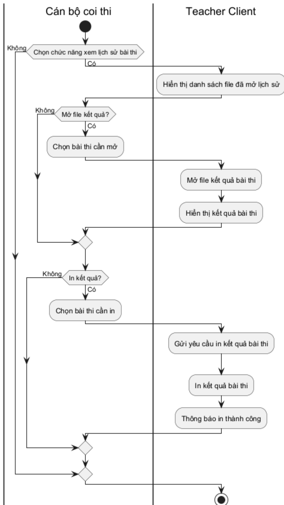
Hình 3.61: Sơ đồ hoạt động cho chức năng lịch sử bài thi thí sinh
