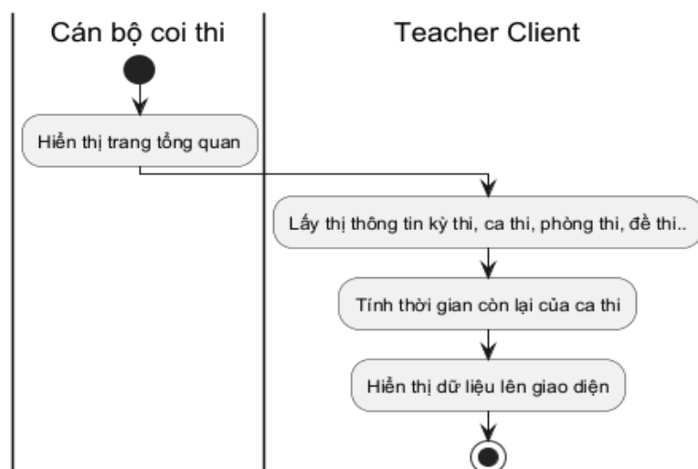
Hình 3.56: Sơ đồ hoạt động cho chức năng tổng quan
