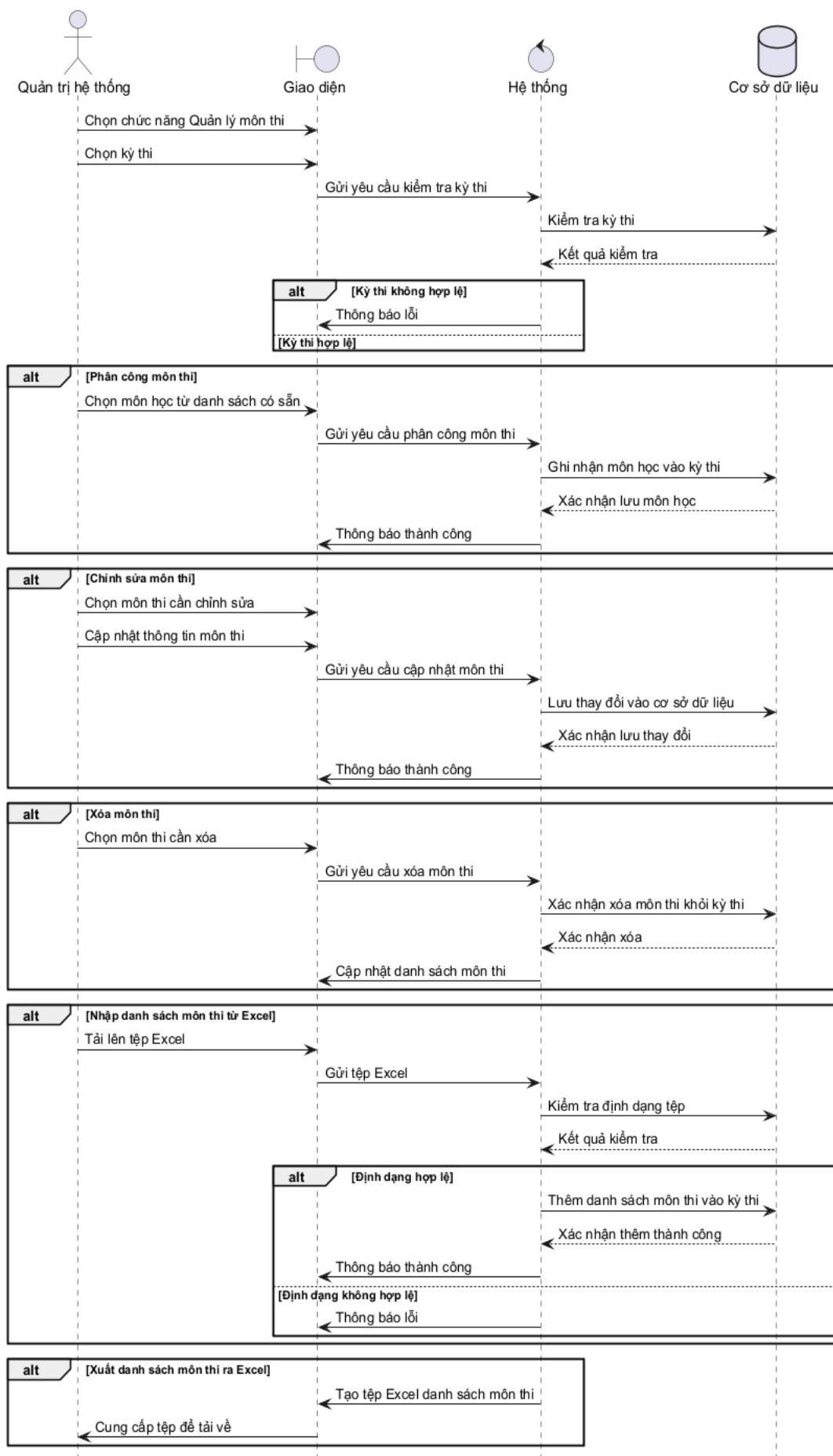
Hình 3.115: Sơ đồ tuần tự cho chức năng quản lý môn thi
