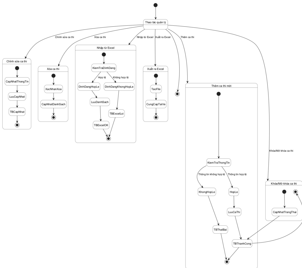
Hình 3.80: Sơ đồ trạng thái cho chức năng quản lý ca thi
