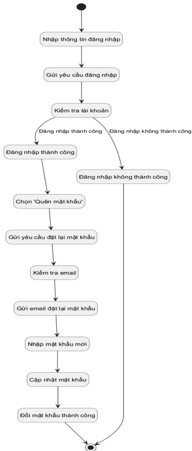
Hình 3.69: Sơ đồ trạng thái cho chức năng đăng nhập
