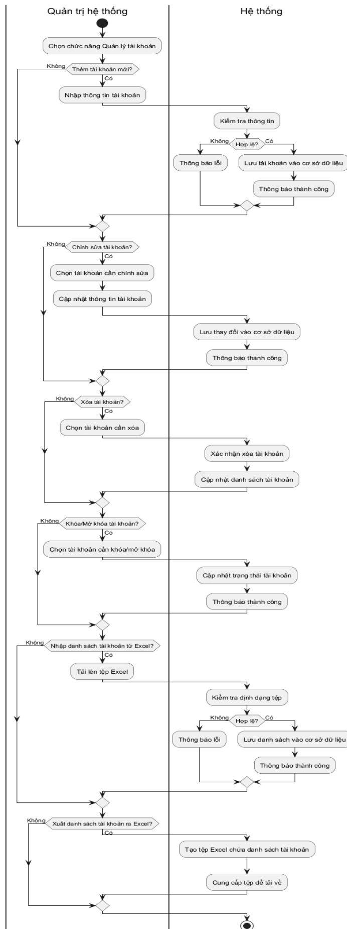
Hình 3.39: Sơ đồ hoạt động cho chức năng quản lý tài khoản
