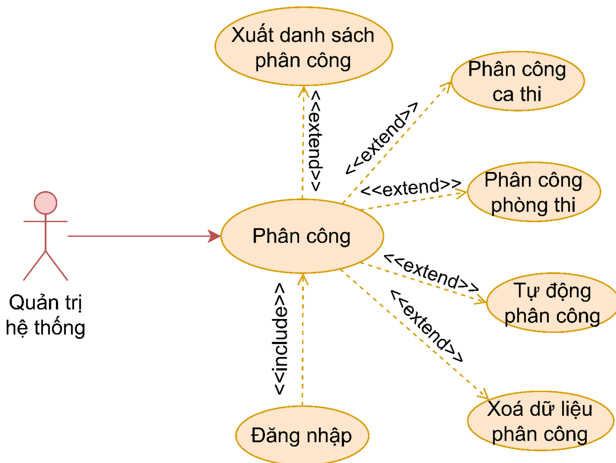
Hình 3.18: Phân rã use case phân công
