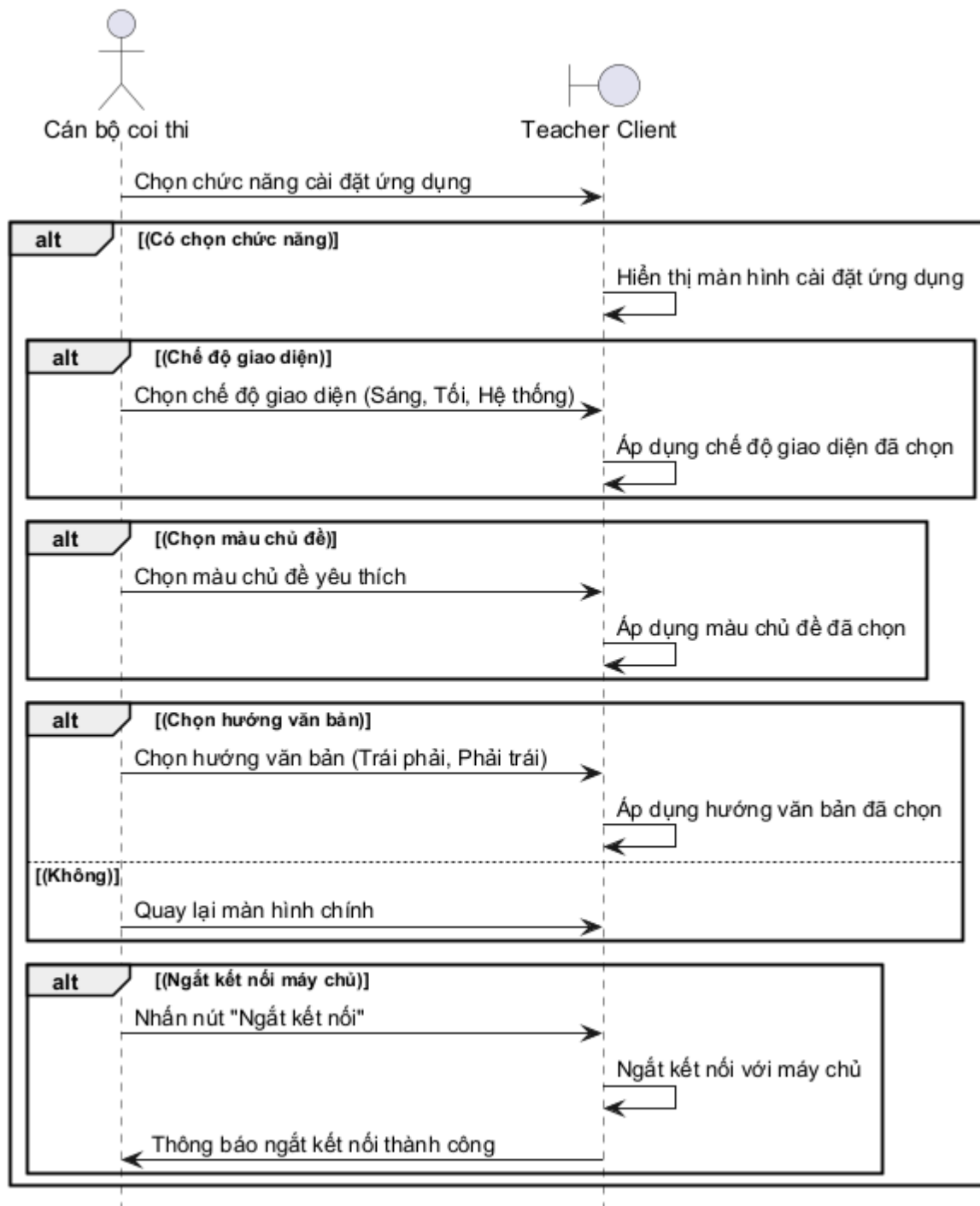
Hình 3.130: Sơ đồ tuần tự cho chức năng cài đặt ứng dụng teacher client
