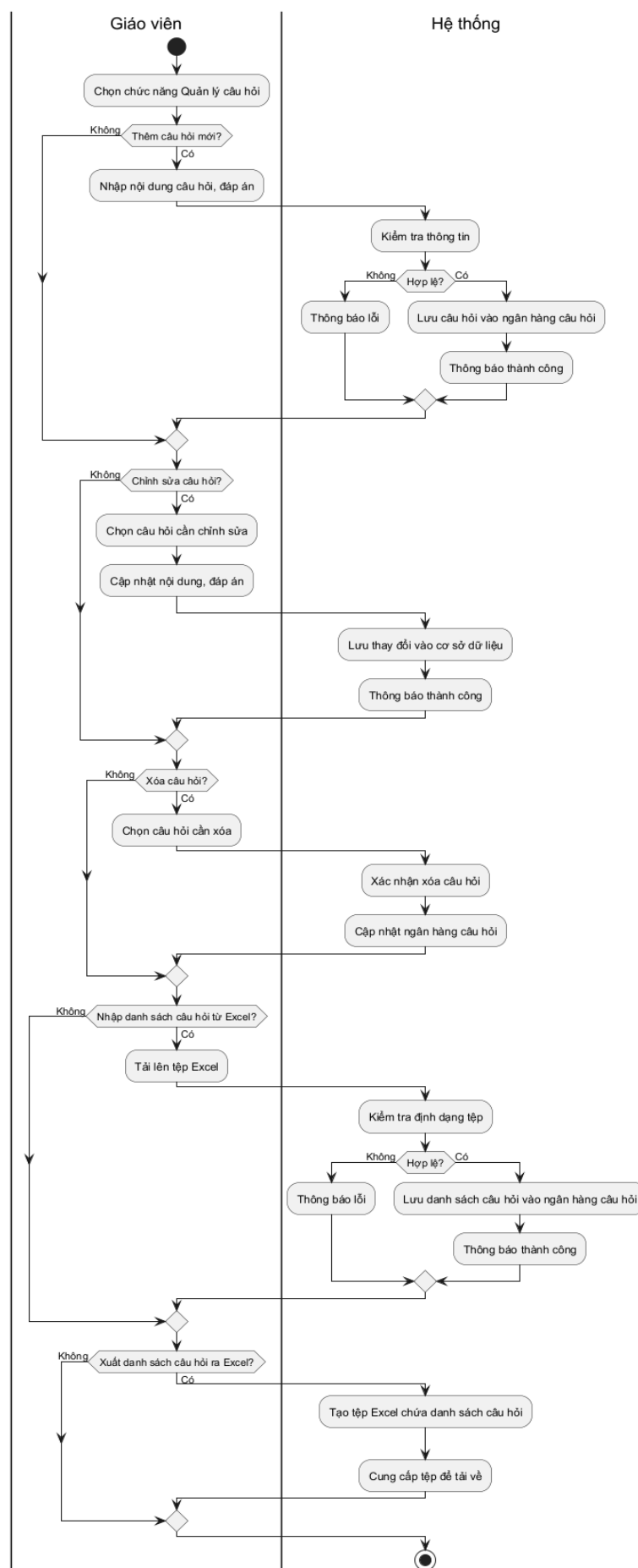
Hình 3.43: Sơ đồ hoạt động cho chức năng quản lý câu hỏi
