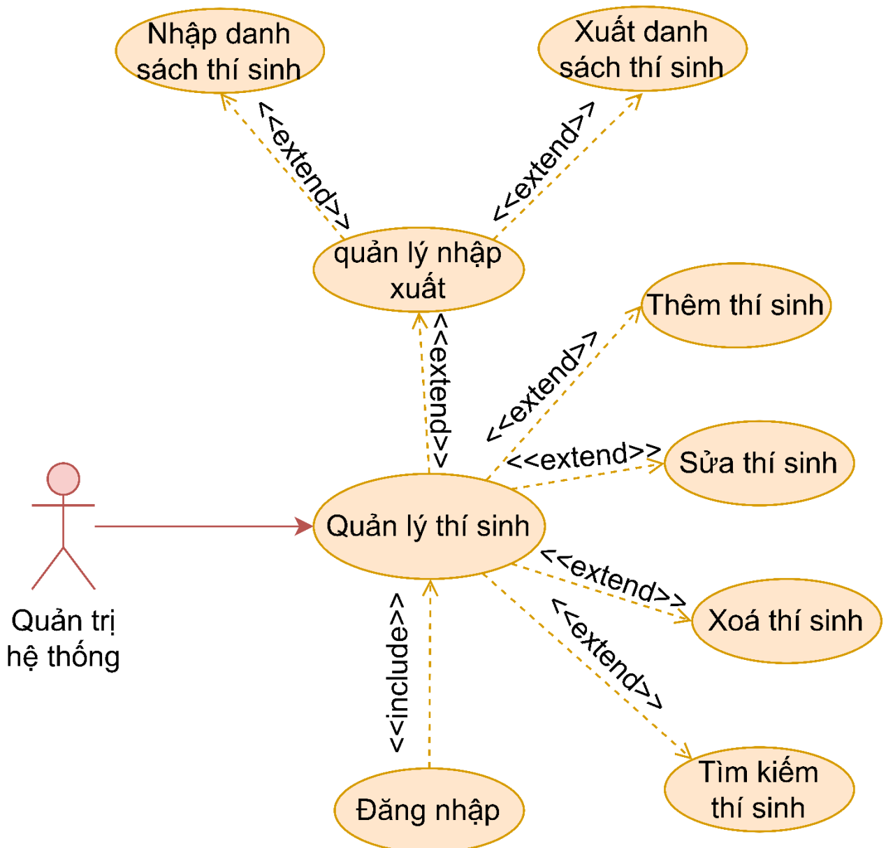
Hình 3.15: Phân rã use case Quản lý thí sinh
