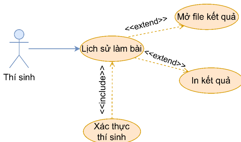
Hình 3.33: Phân rã use case Lịch sử làm bài
