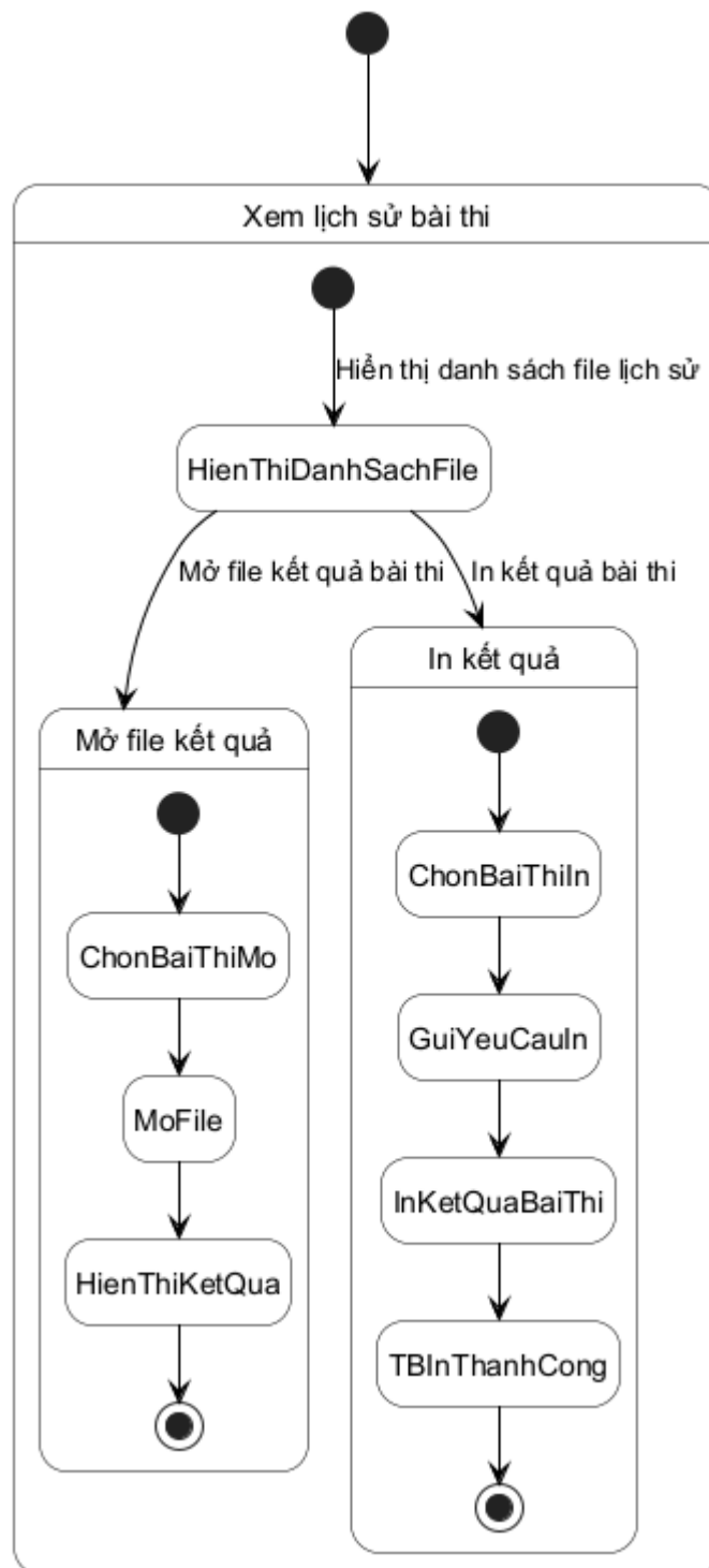
Hình 3.95: Sơ đồ trạng thái cho chức năng lịch sử bài thi thí sinh
