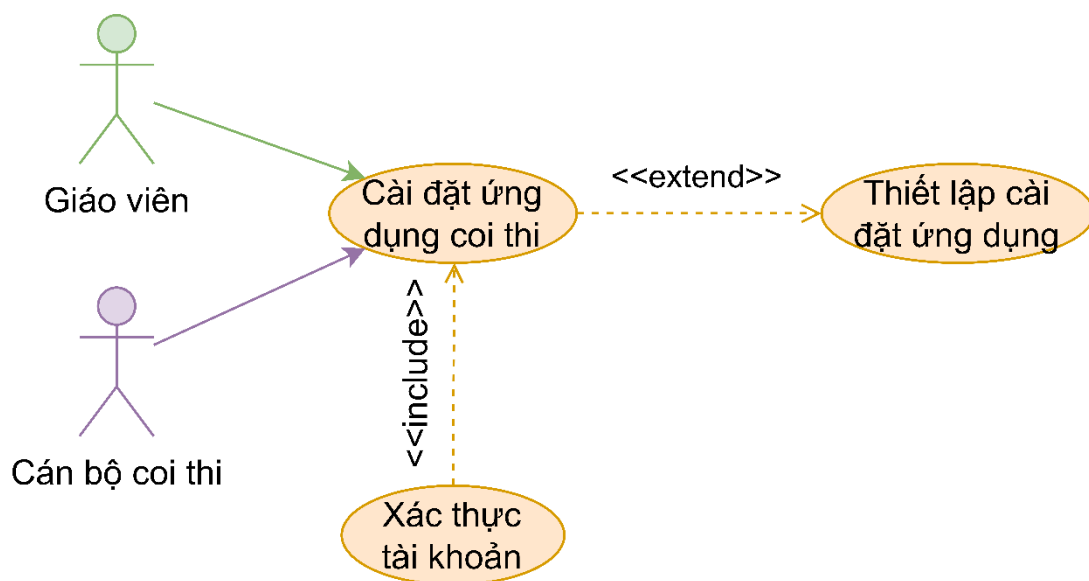
Hình 3.28: Phân rã use case cài đặt ứng dụng coi thi
