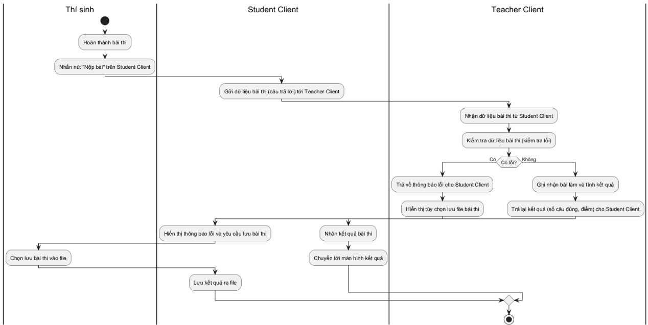
Hình 3.66: Sơ đồ hoạt động cho chức năng làm bài
