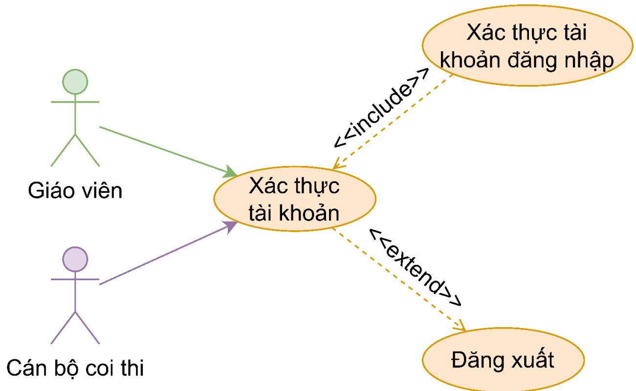
Hình 3.22: Phân rã use case Xác thực tài khoản
