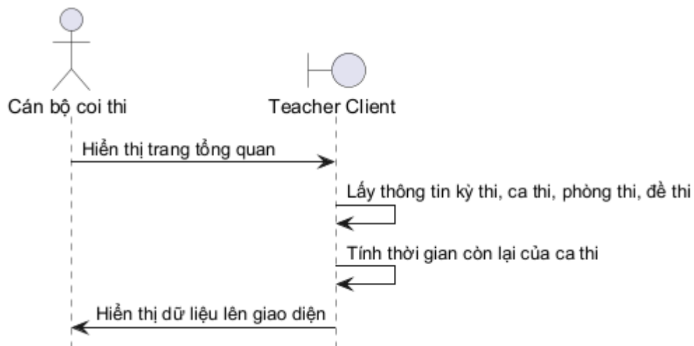
Hình 3.124: Sơ đồ tuần tự cho chức năng tổng quan
