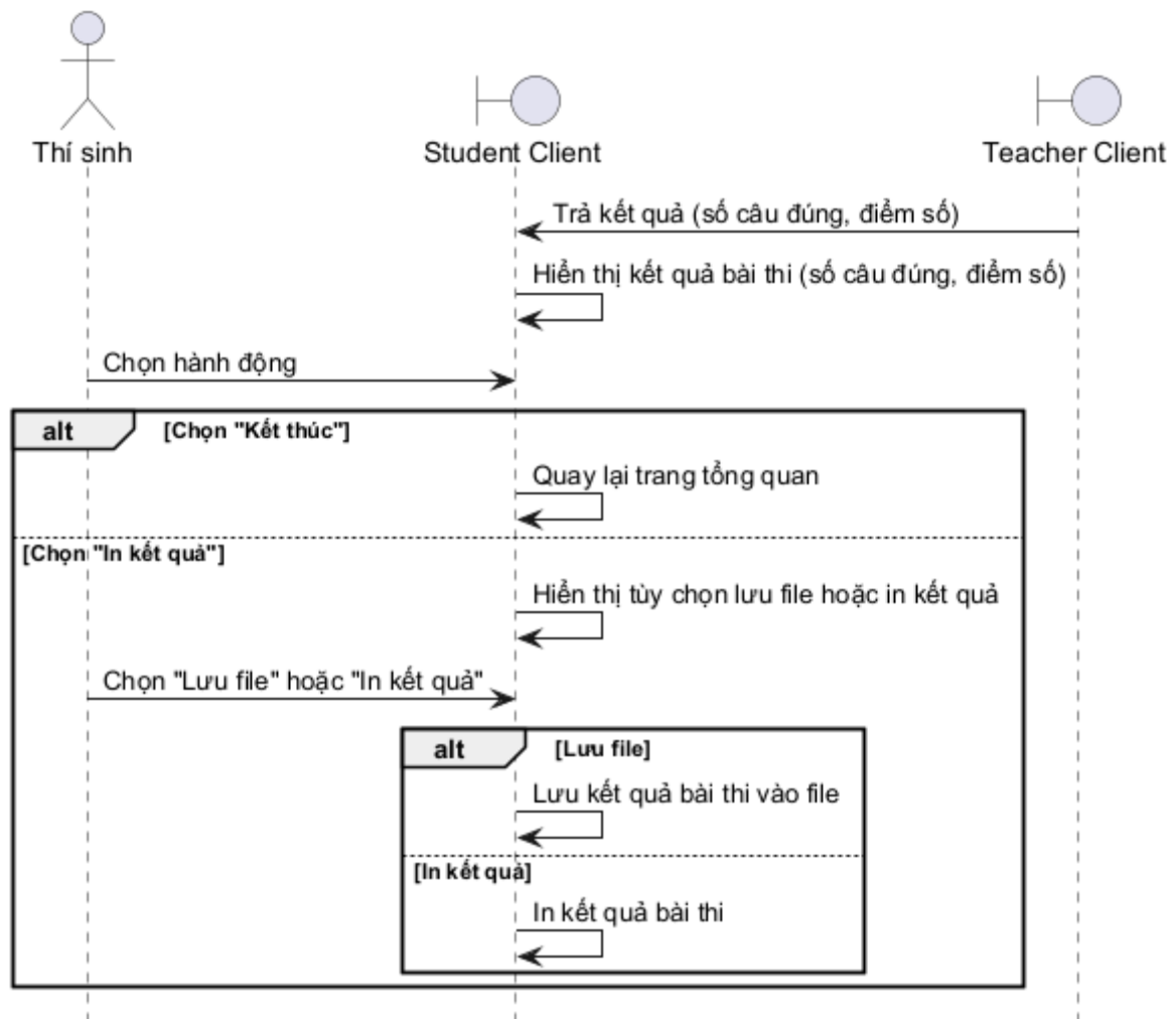
Hình 3.135: Sơ đồ tuần tự cho chức năng kết quả
