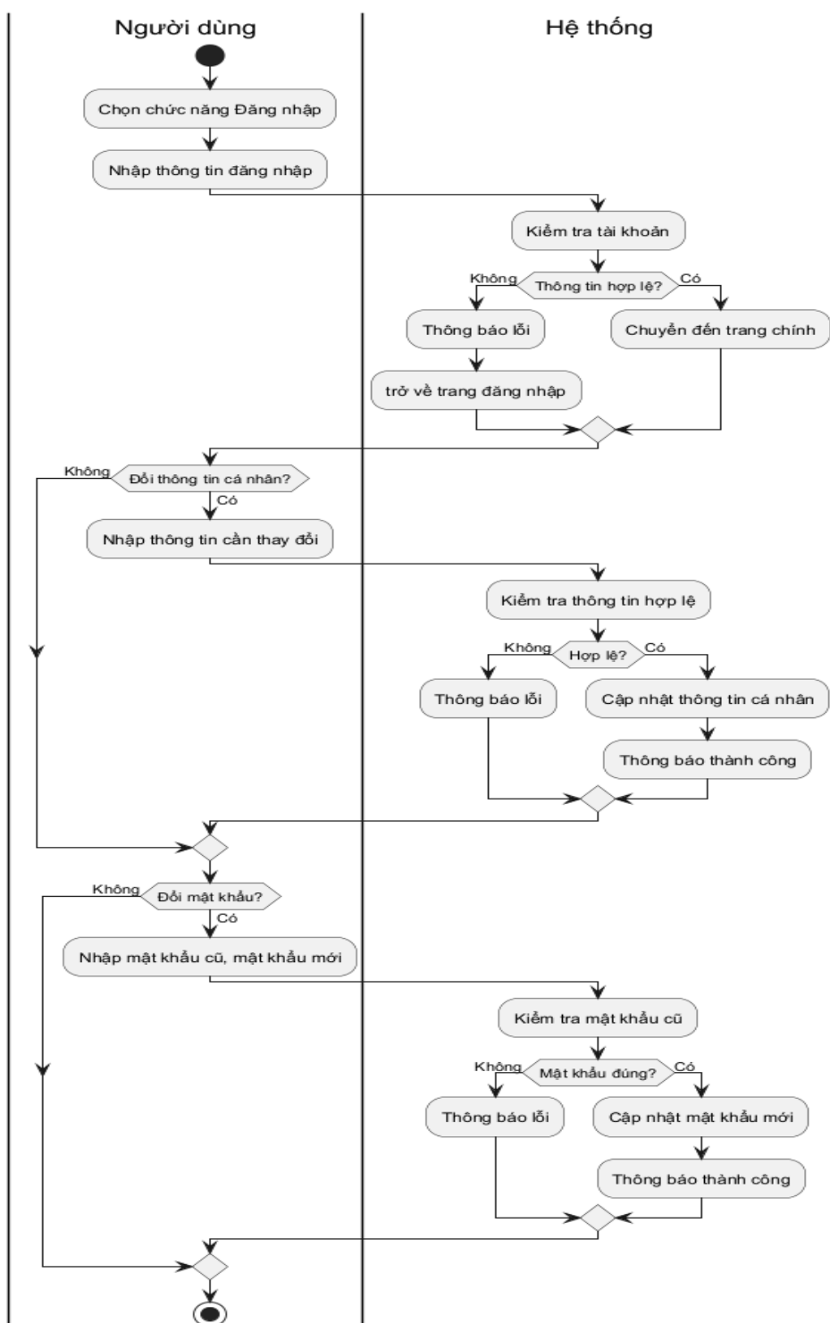
Hình 3.35: Sơ đồ hoạt động cho chức năng đăng nhập
