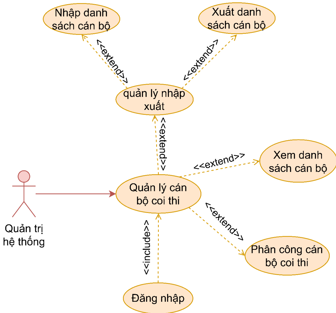
Hình 3.16: Phân rã use case quản lý cán bộ coi thi
