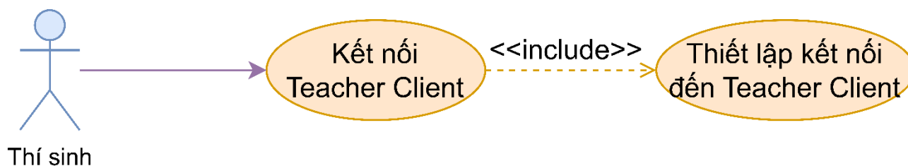
Hình 3.29: Phân rã use case Kết nối Teacher client
