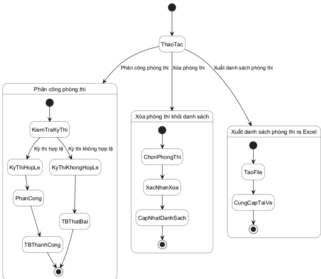
Hình 3.84: Sơ đồ trạng thái cho chức năng quản lý phòng thi thuộc kỳ thi
