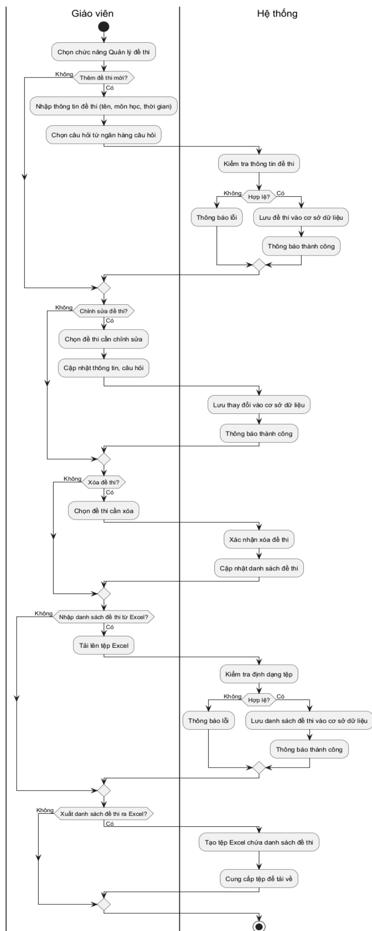
Hình 3.44: Sơ đồ hoạt động cho chức năng quản lý đề thi
