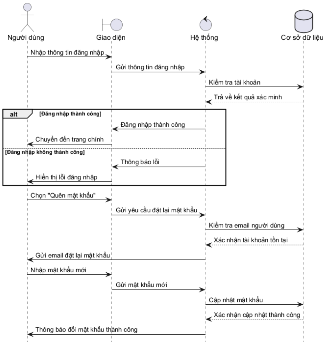
Hình 3.103: Sơ đồ tuần tự cho chức năng Đăng nhập
