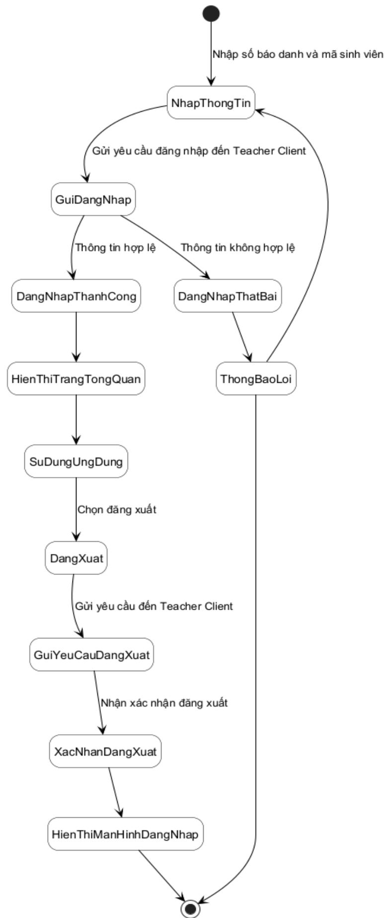
Hình 3.98: Sơ đồ trạng thái cho chức năng xác thực thí sinh
