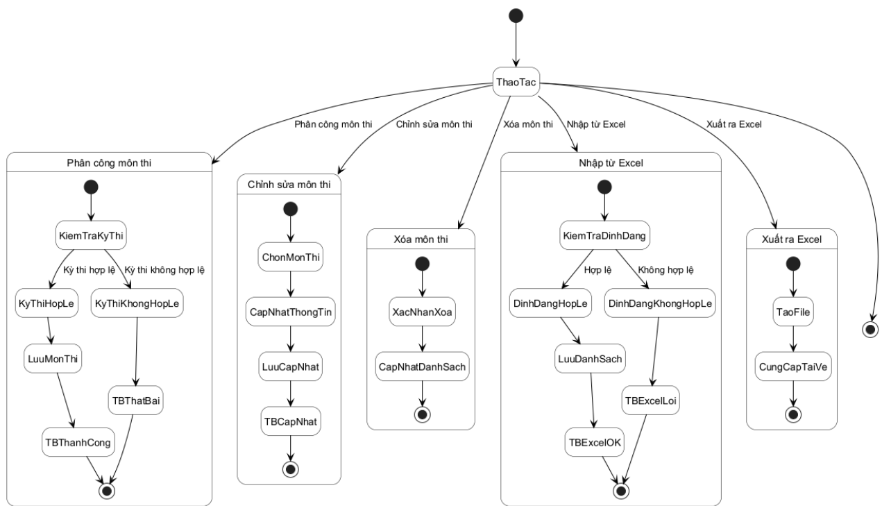
Hình 3.81: Sơ đồ trạng thái cho chức năng quản lý môn thi
