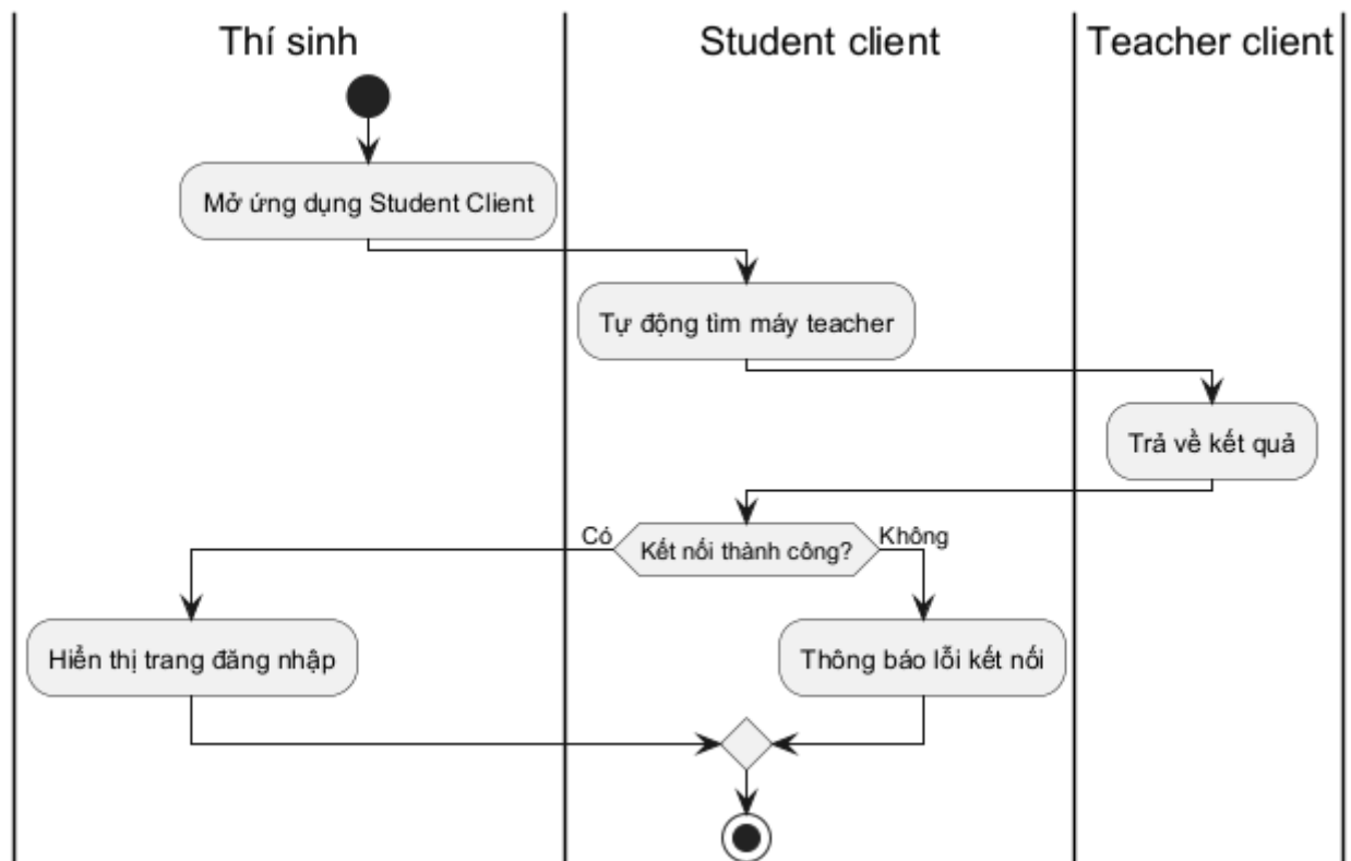
Hình 3.63: Sơ đồ hoạt động cho chức năng kết nối teacher client
