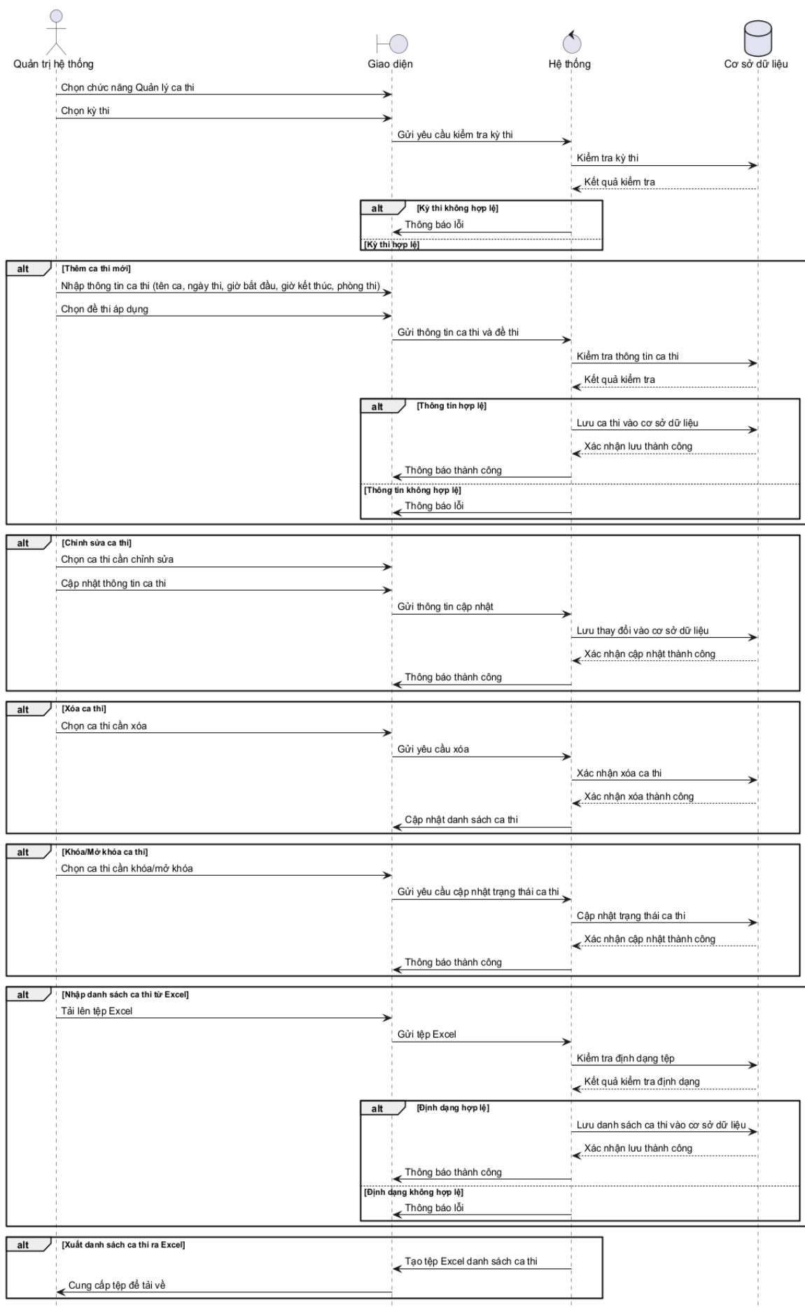
Hình 3.114: Sơ đồ tuần tự cho chức năng quản lý ca thi
