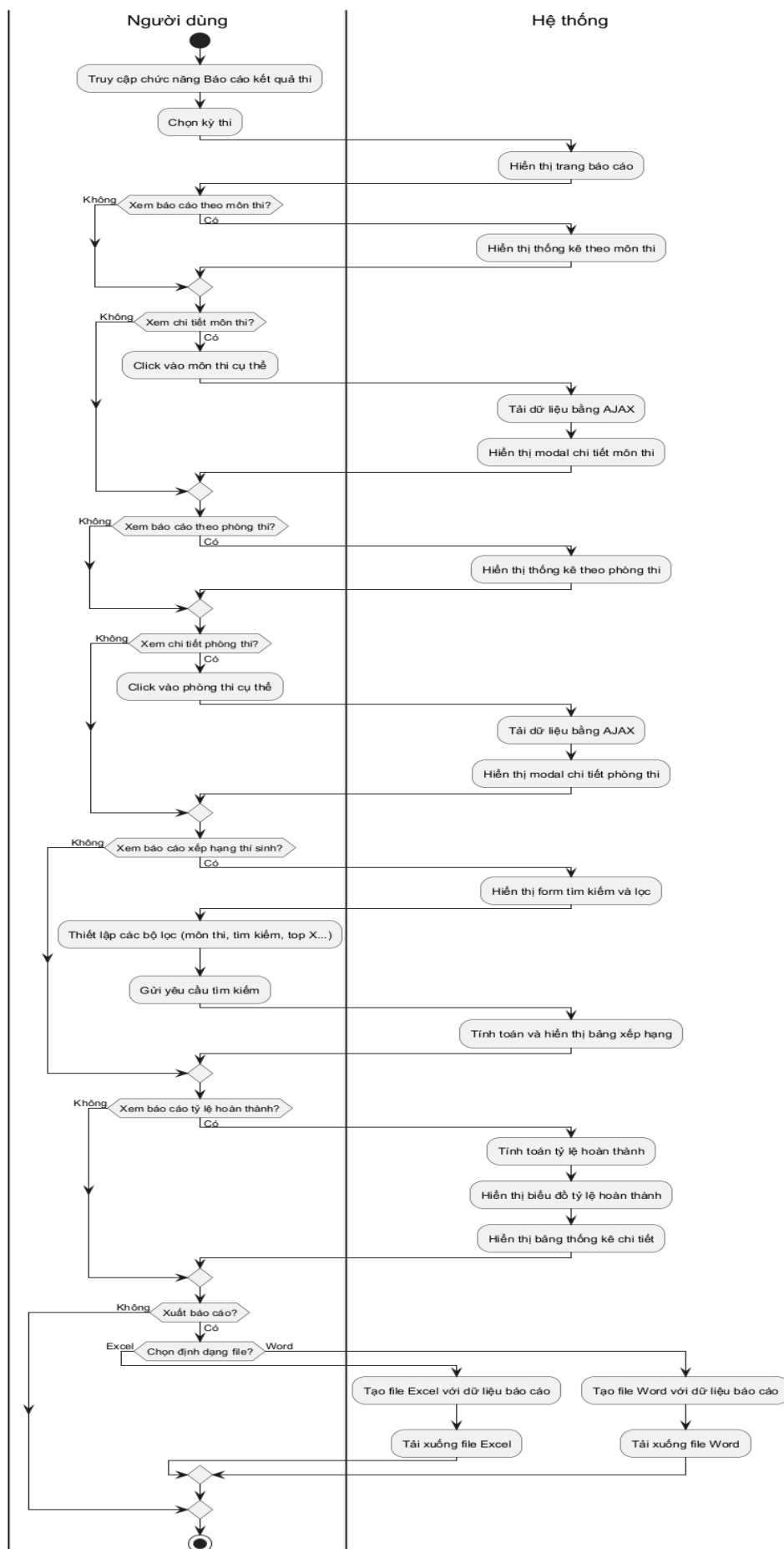
Hình 3.53: Sơ đồ hoạt động cho chức năng báo cáo thống kê
