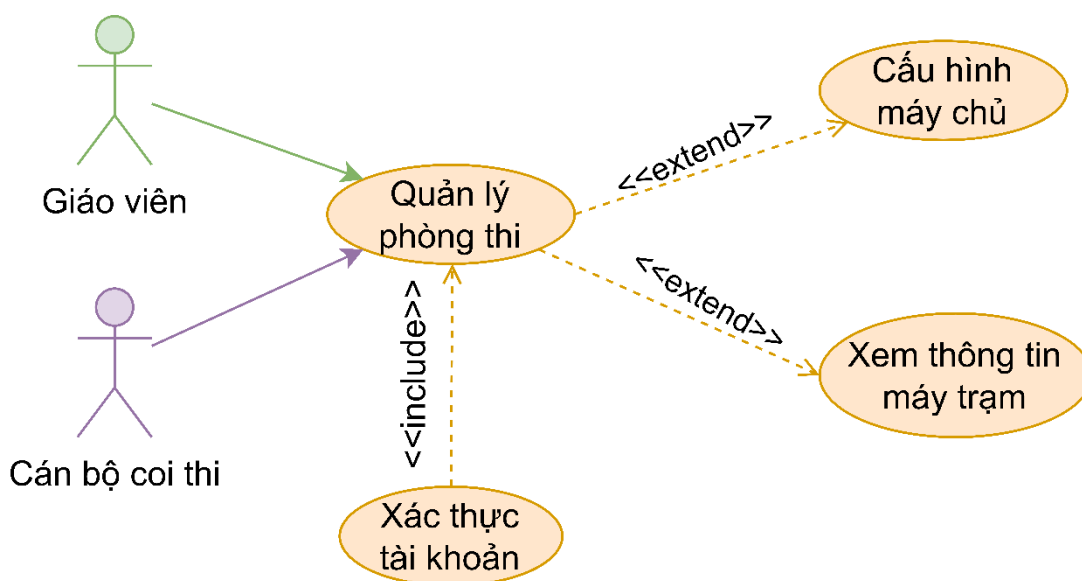
Hình 3.25: Phân rã use case quản lý phòng thi
