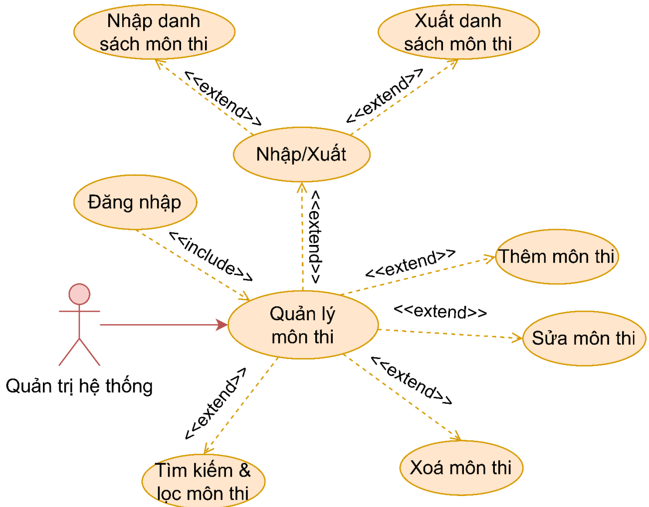
Hình 3.14: Phân rã use case Quản lý môn thi
