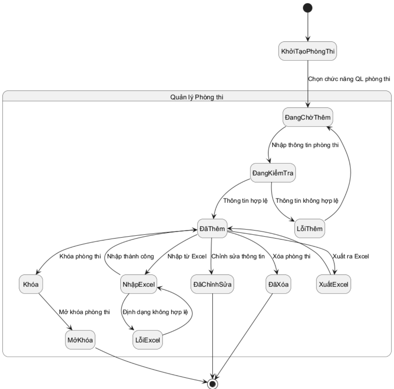
Hình 3.72: Sơ đồ trạng thái cho chức năng quản lý phòng thi
