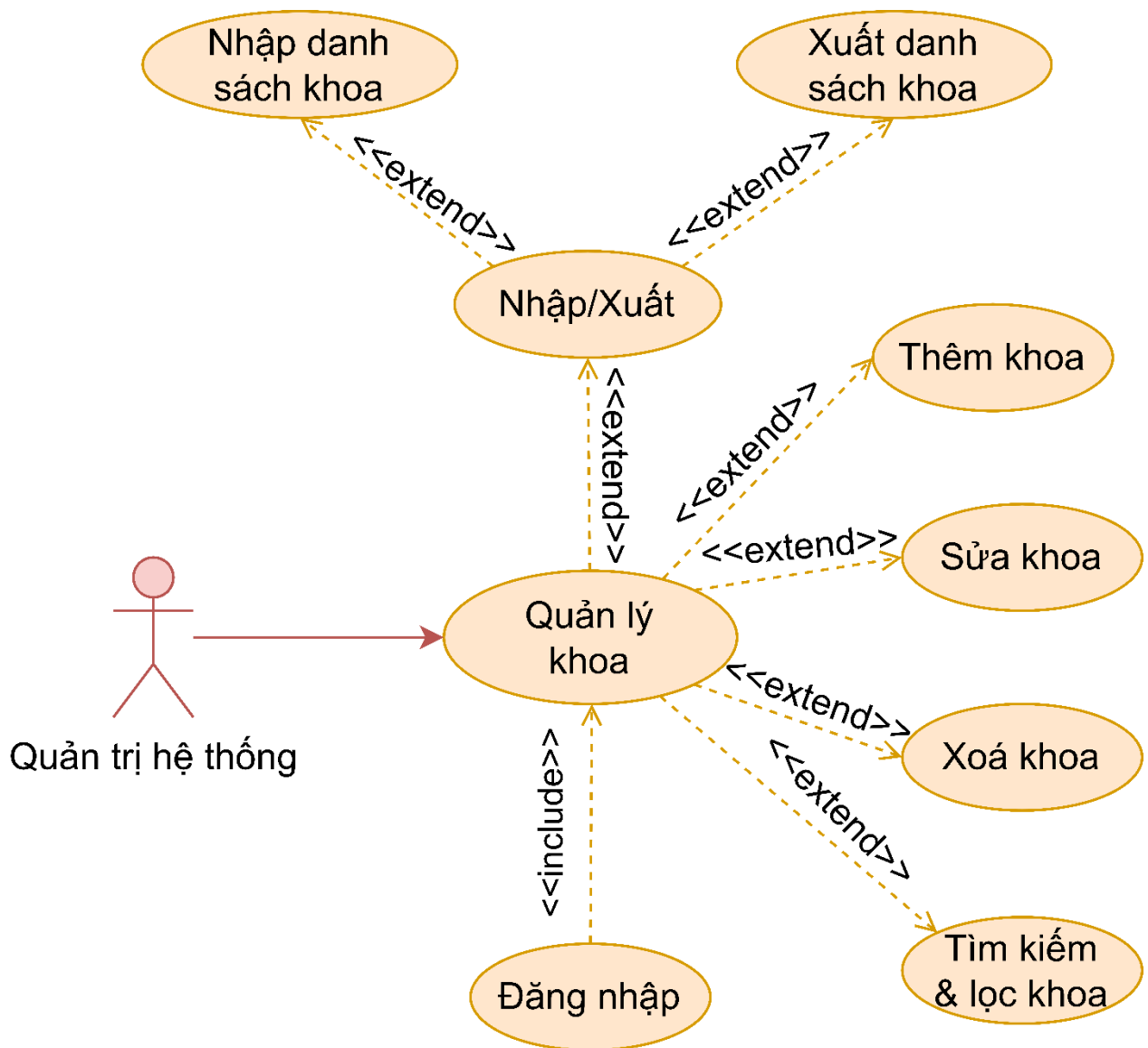
Hình 3.6: Phân rã use case Quản lý khoa
