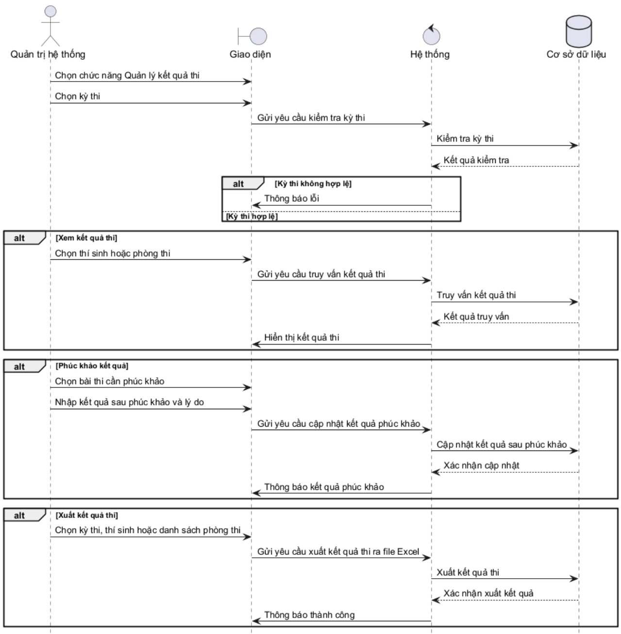
Hình 3.120: Sơ đồ tuần tự cho chức năng quản lý kết quả thi
