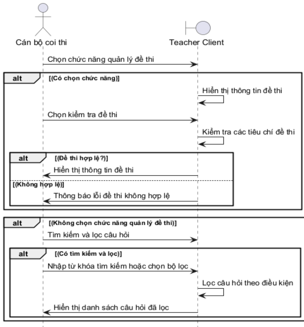
Hình 3.124: Sơ đồ tuần tự cho chức năng tổng quan
