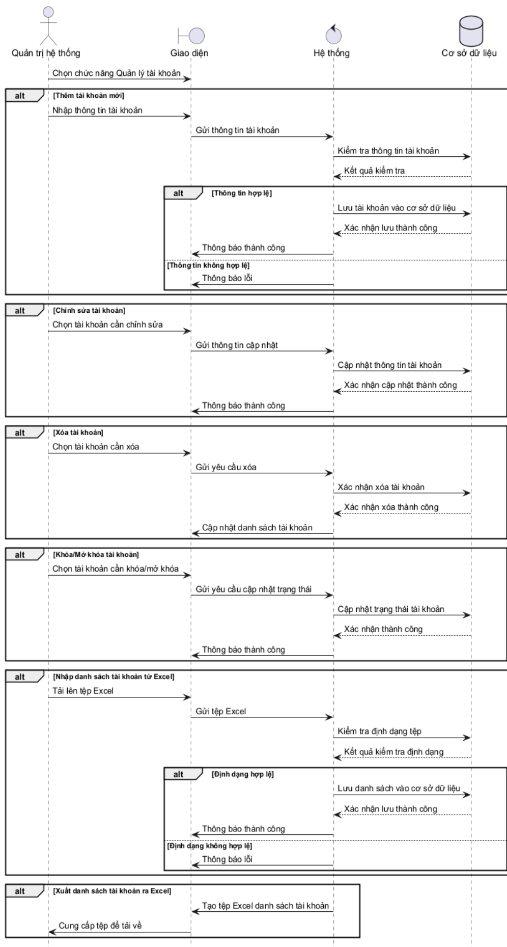
Hình 3.107: Sơ đồ tuần tự cho chức năng quản lý tài khoản
