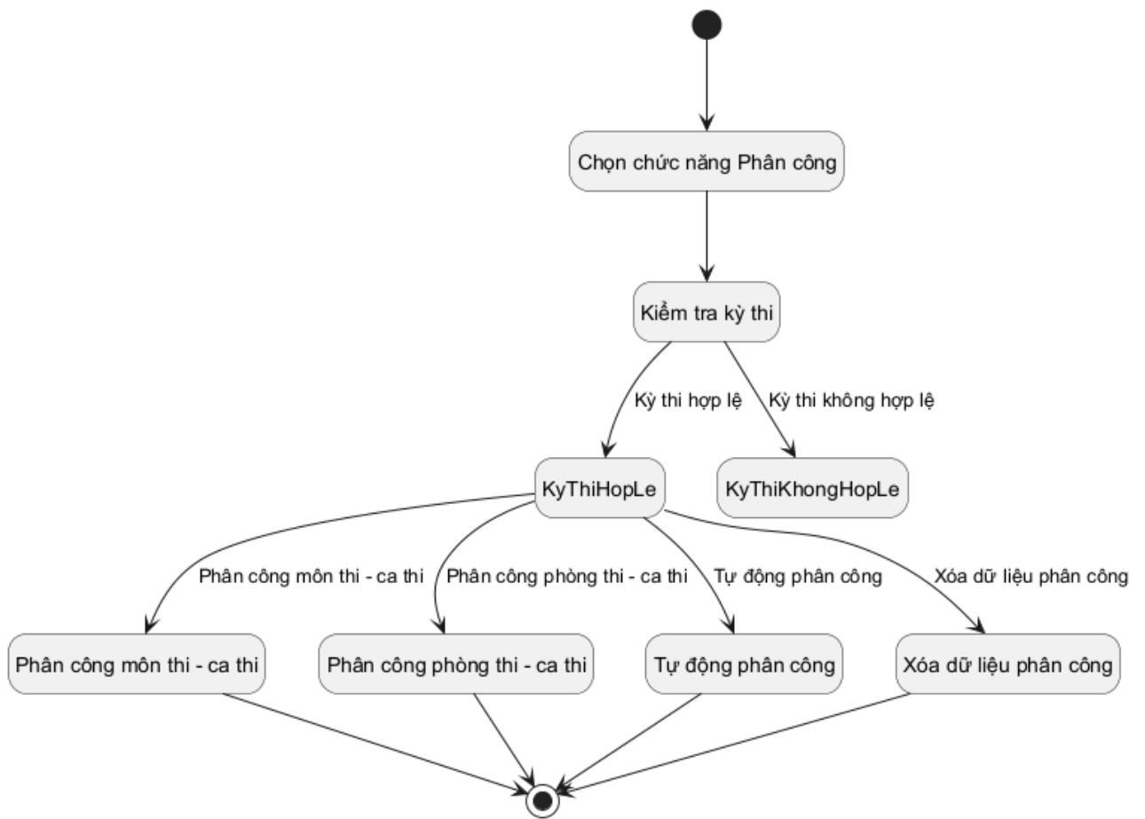
Hình 3.85: Sơ đồ trạng thái cho chức năng phân công
