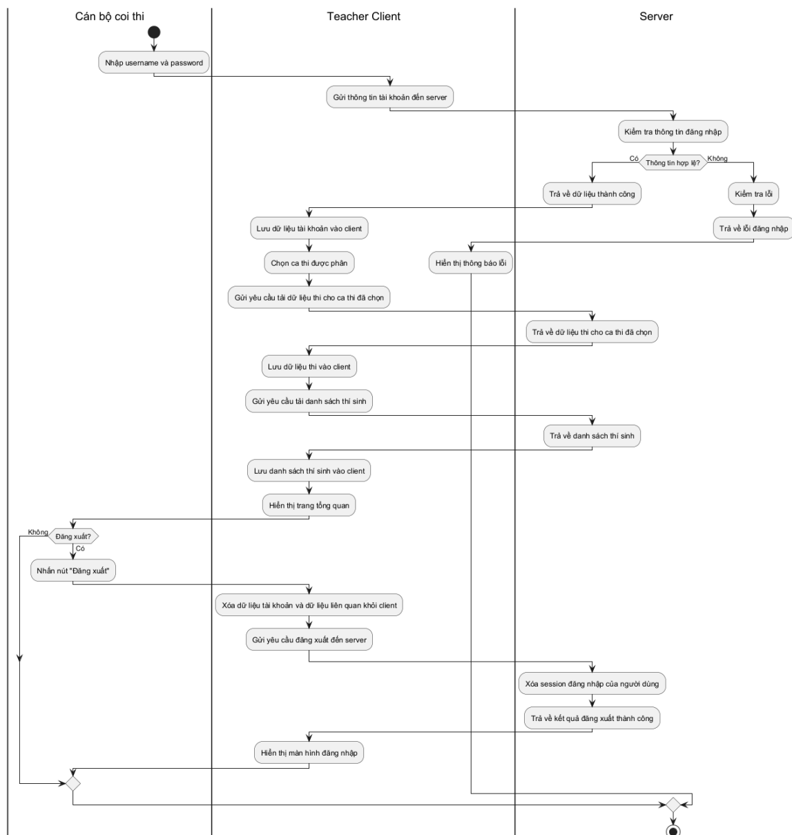
Hình 3.55: Sơ đồ hoạt động cho chức năng xác thực tài khoản
