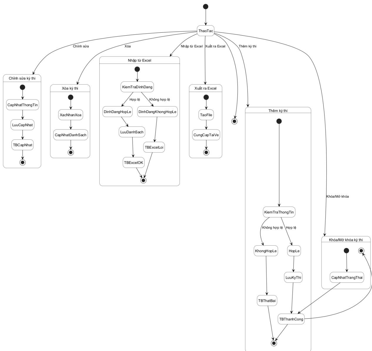
Hình 3.79: Sơ đồ trạng thái cho chức năng quản lý kỳ thi
