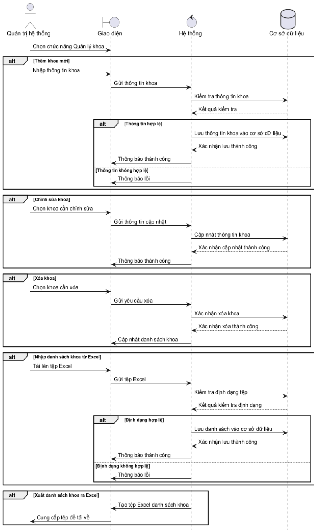
Hình 3.108: Sơ đồ tuần tự cho chức năng quản lý khoa
