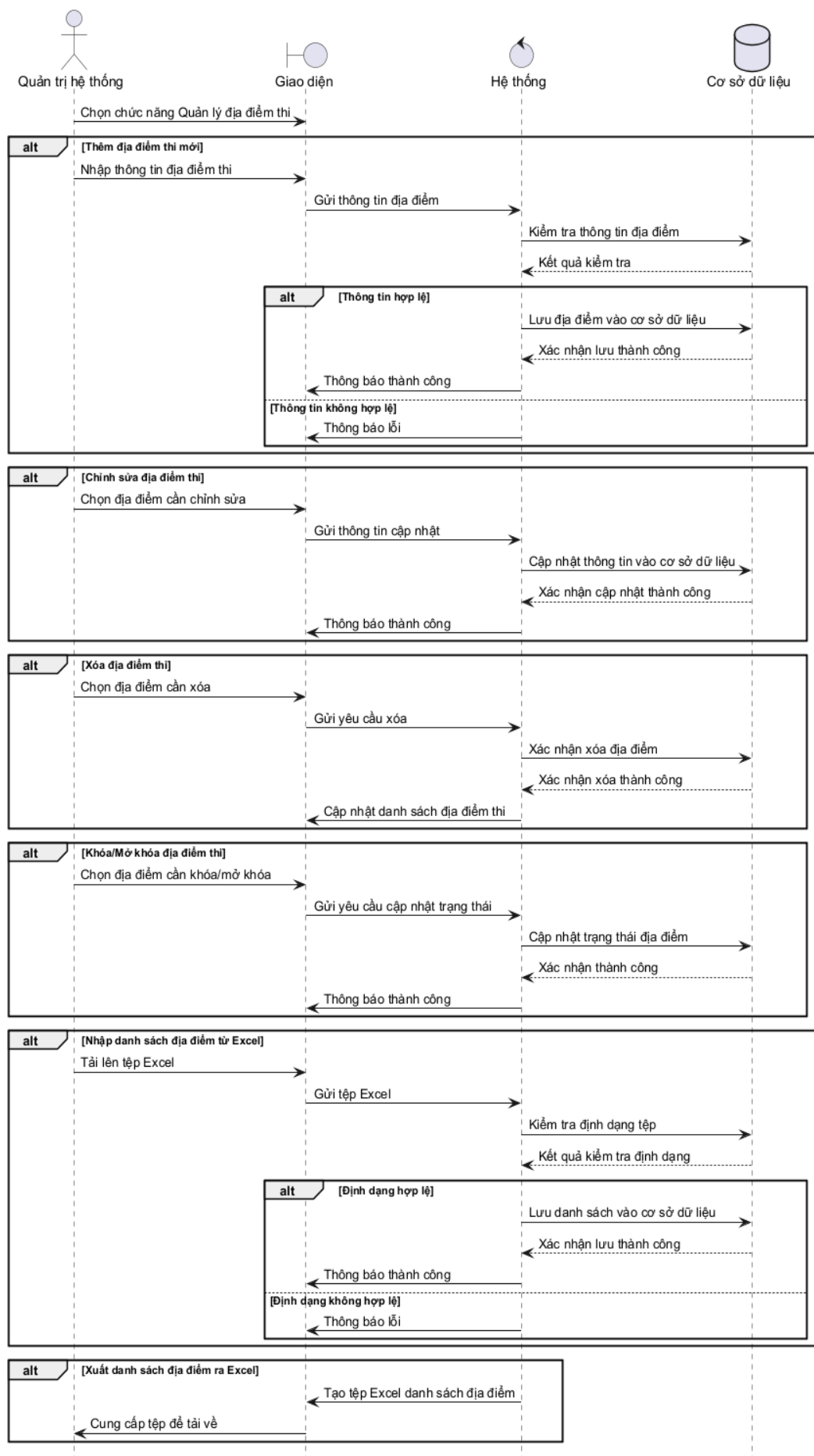
Hình 3.105: Sơ đồ tuần tự cho chức năng quản lý địa điểm thi
