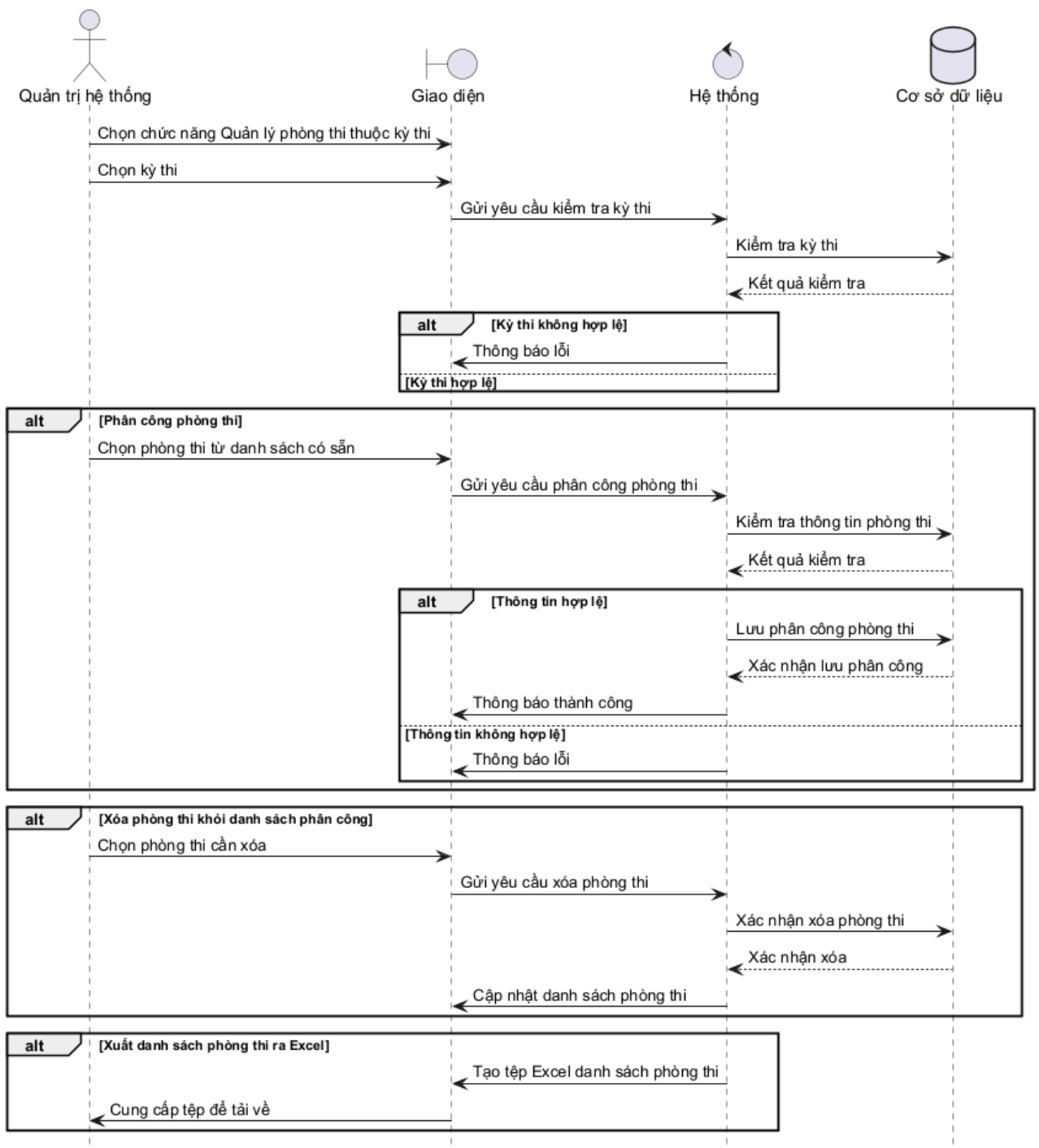
Hình 3.118: Sơ đồ tuần tự cho chức năng quản lý phòng thi thuộc kỳ thi
