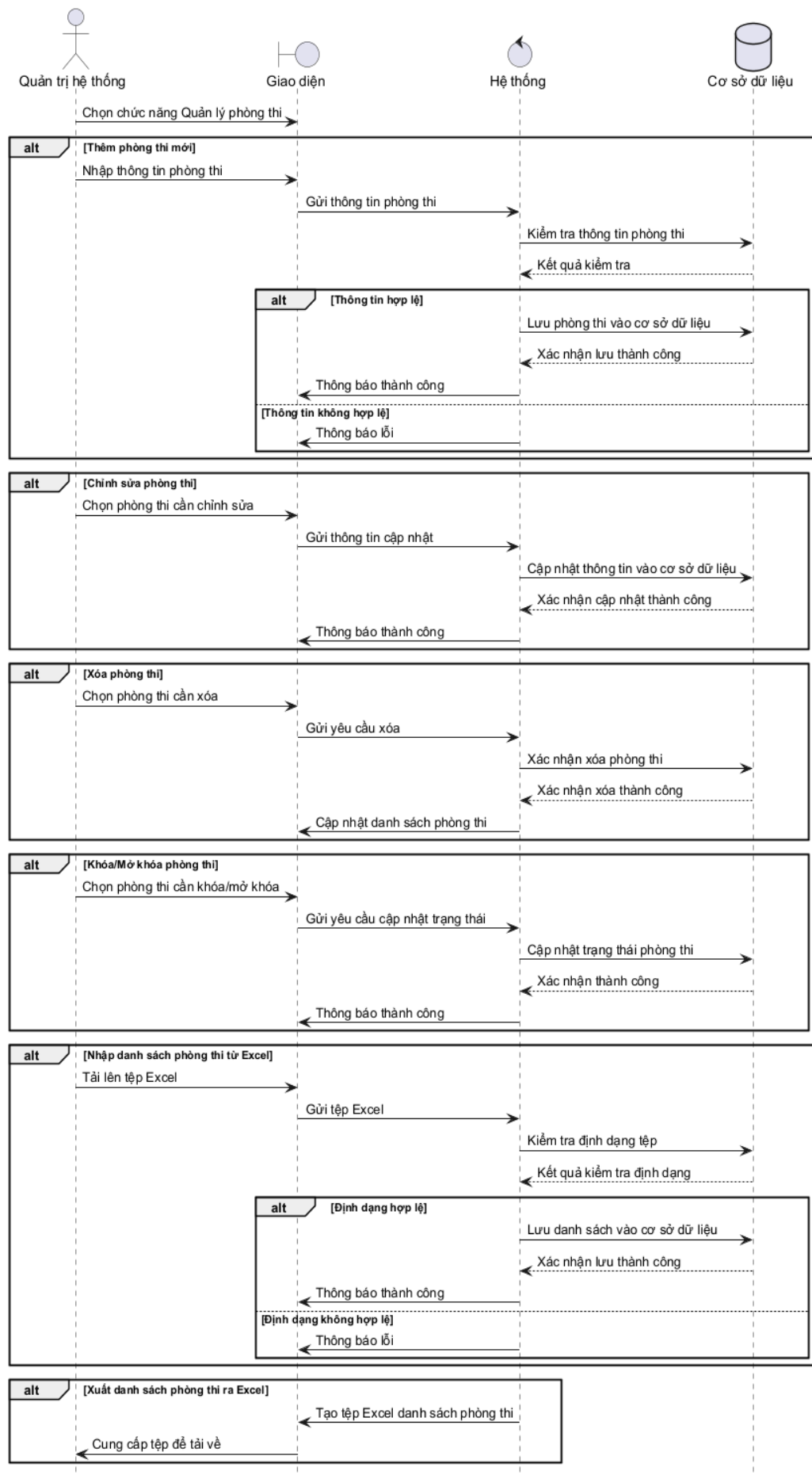
Hình 3.106: Sơ đồ tuần tự cho chức năng quản lý phòng thi
