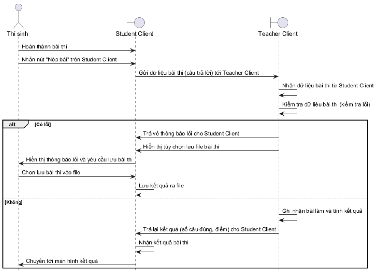
Hình 3.133: Sơ đồ tuần tự cho chức năng tổng quan bài thi
