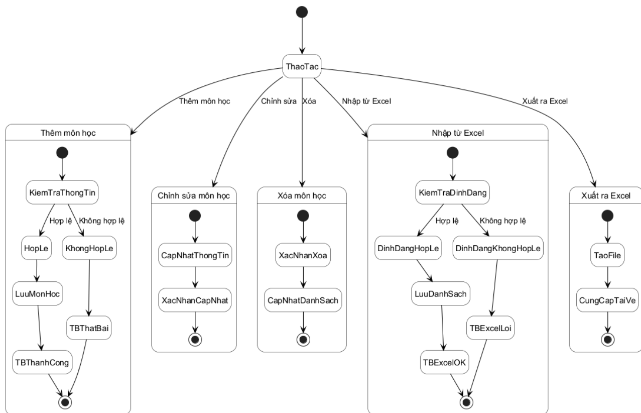
Hình 3.76: Sơ đồ trạng thái cho chức năng quản lý môn học
