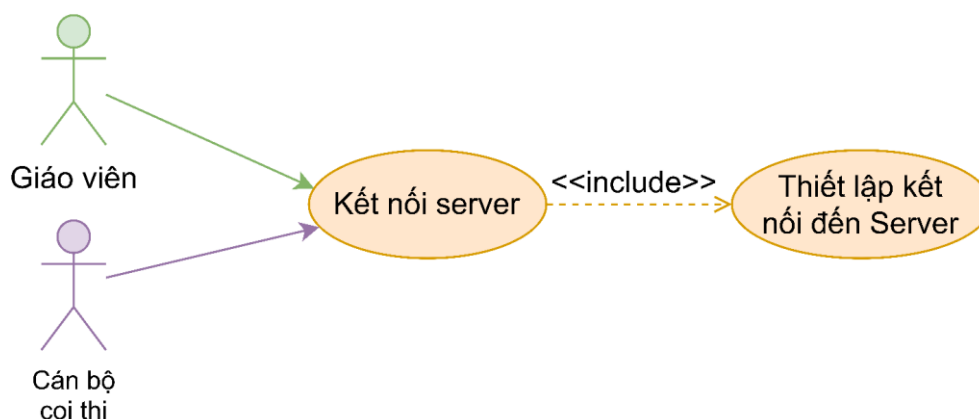
Hình 3.21: Phân rã use case kết nối Server
