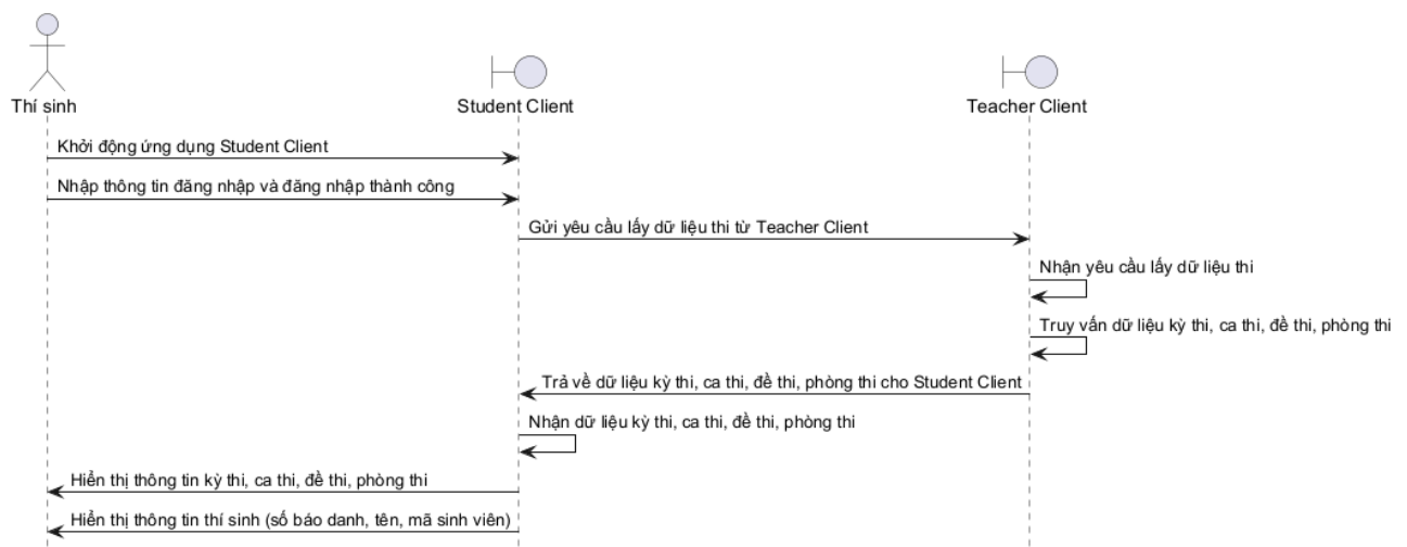
Hình 3.133: Sơ đồ tuần tự cho chức năng tổng quan bài thi
