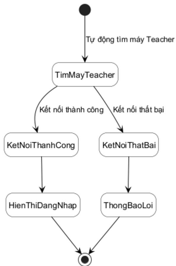
Hình 3.97: Sơ đồ trạng thái cho chức năng kết nối teacher client
