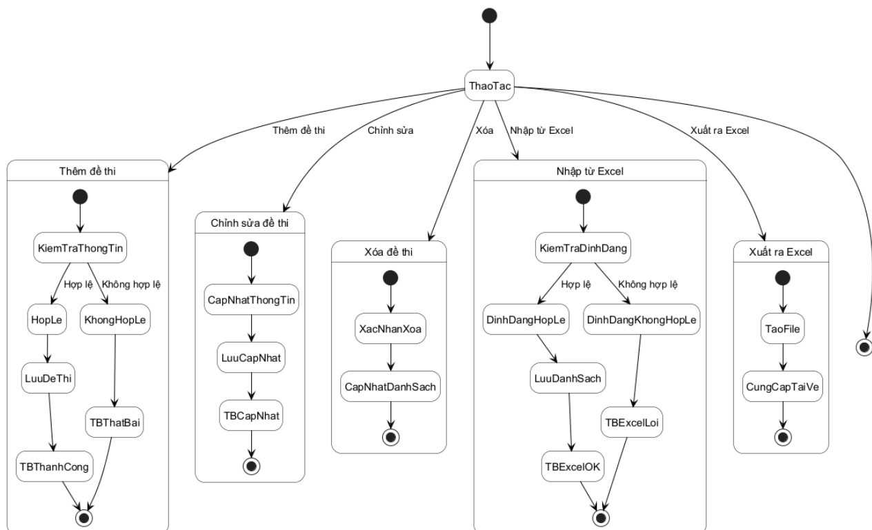
Hình 3.78: Sơ đồ trạng thái cho chức năng quản lý đề thi
