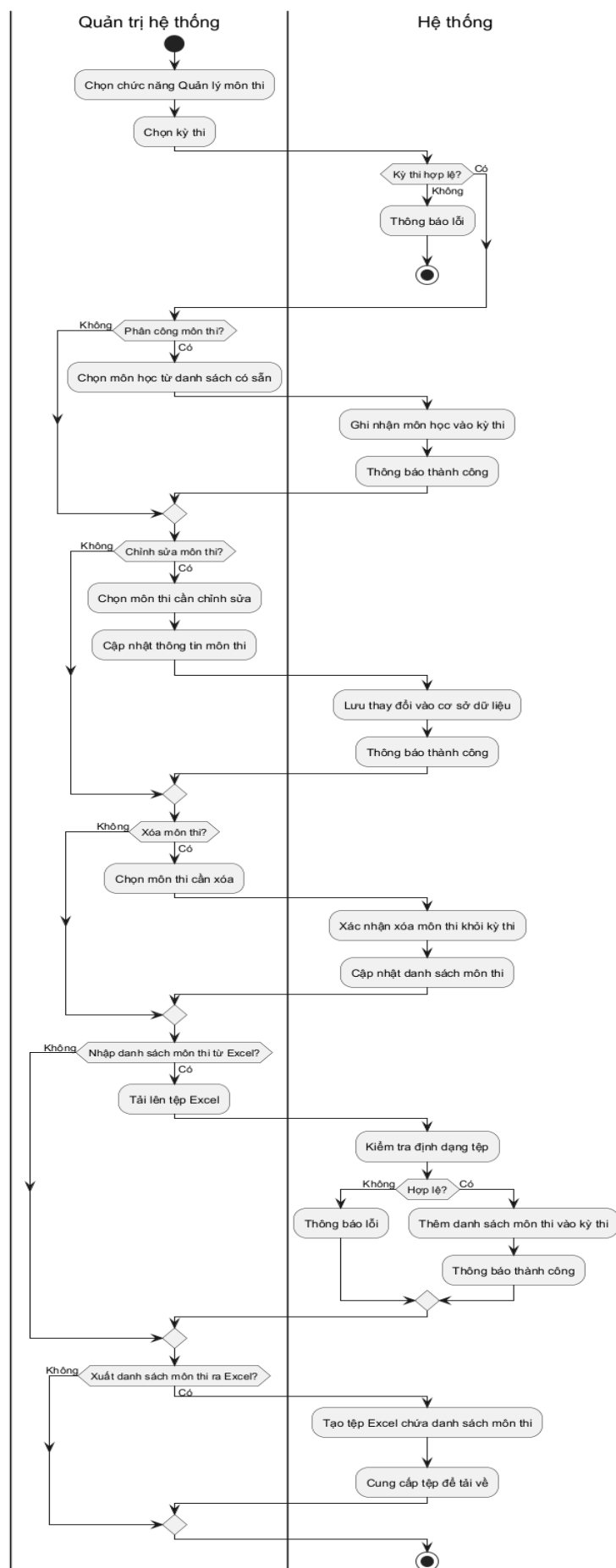
Hình 3.47: Sơ đồ hoạt động cho chức năng quản lý môn thi
