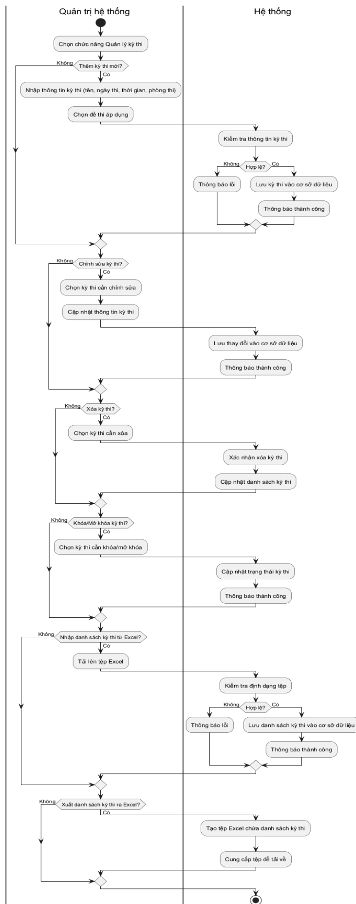
Hình 3.45: Sơ đồ hoạt động cho chức năng quản lý kỳ thi
