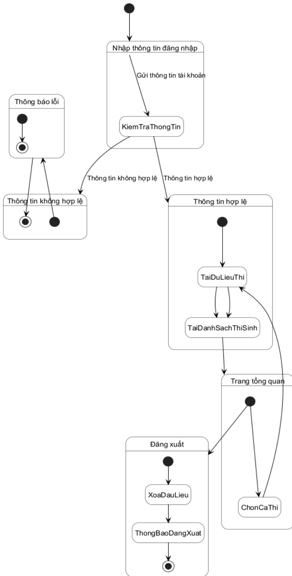
Hình 3.89: Sơ đồ trạng thái cho chức năng xác thực tài khoản
