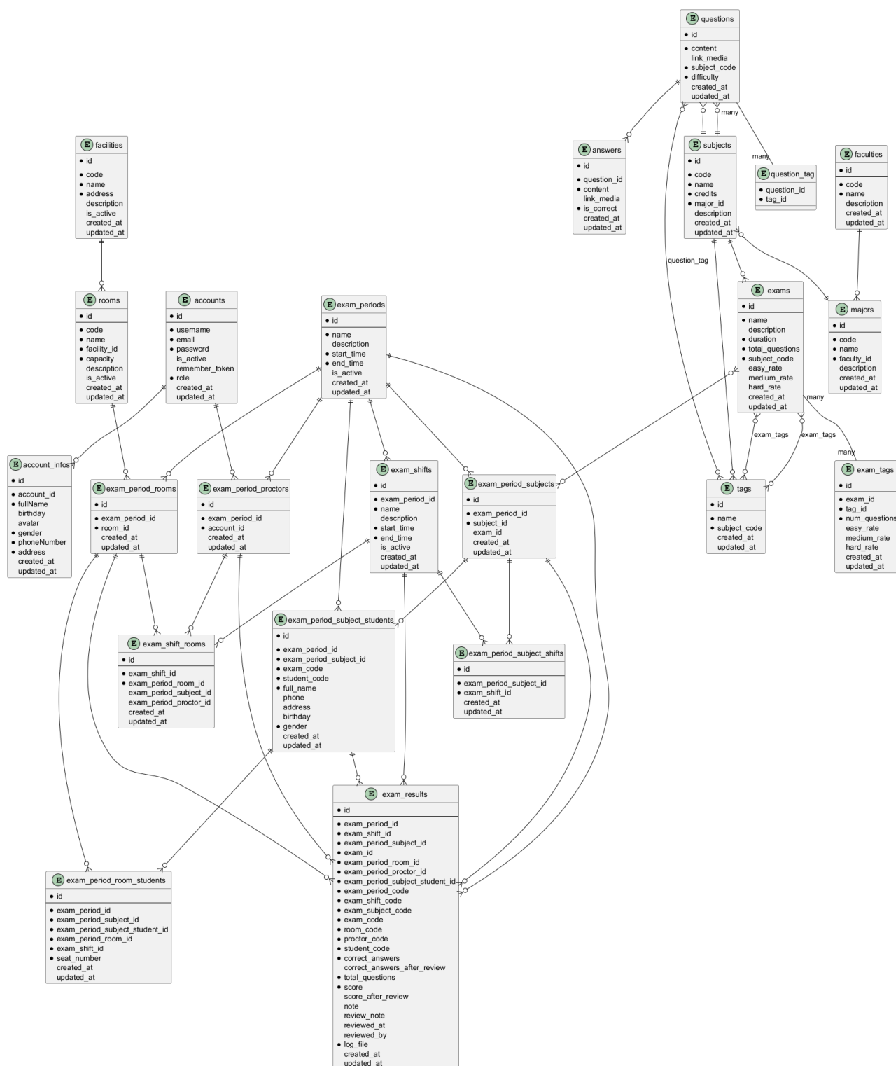
Hình 3.139: Mô hình quan hệ
