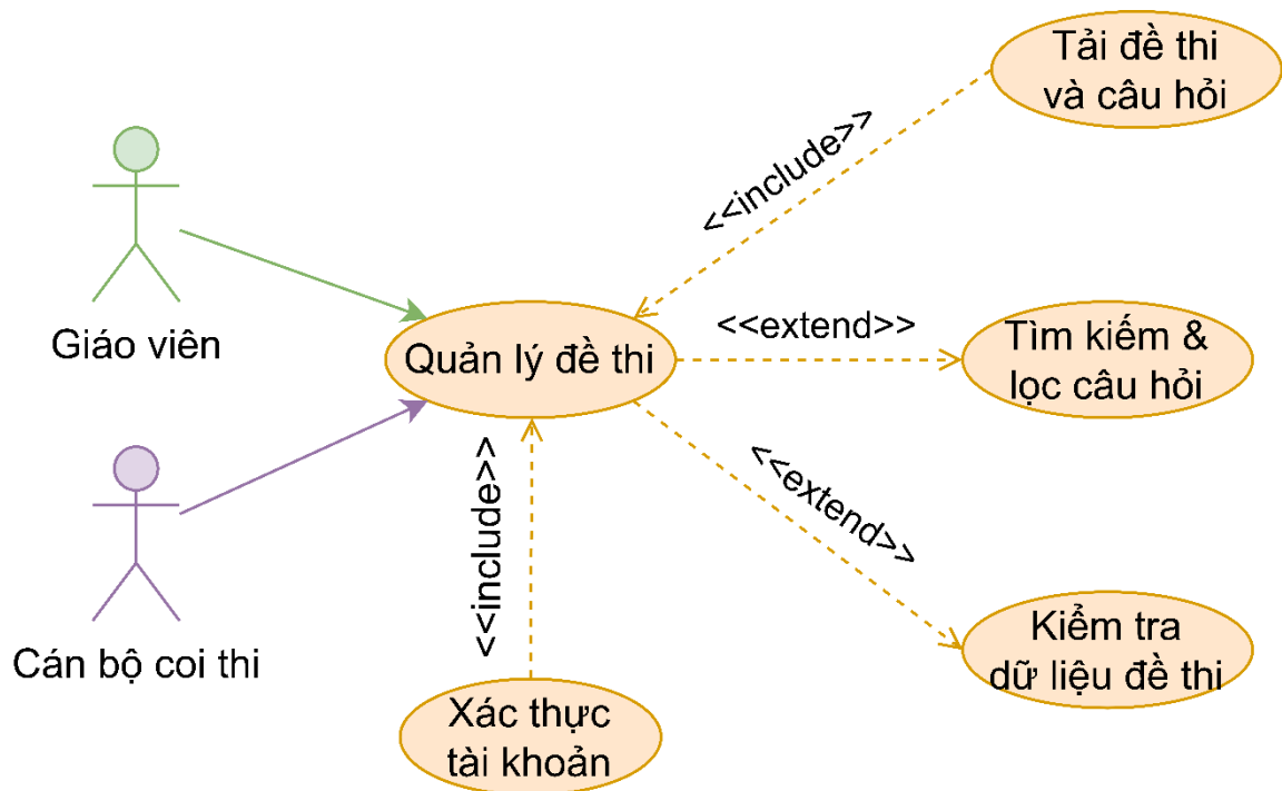
Hình 3.23: Phân rã use case quản lý đề thi
