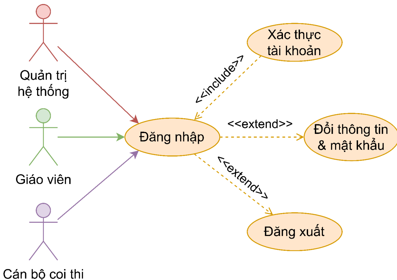
Hình 3.2: Phân rã use case Đăng nhập
