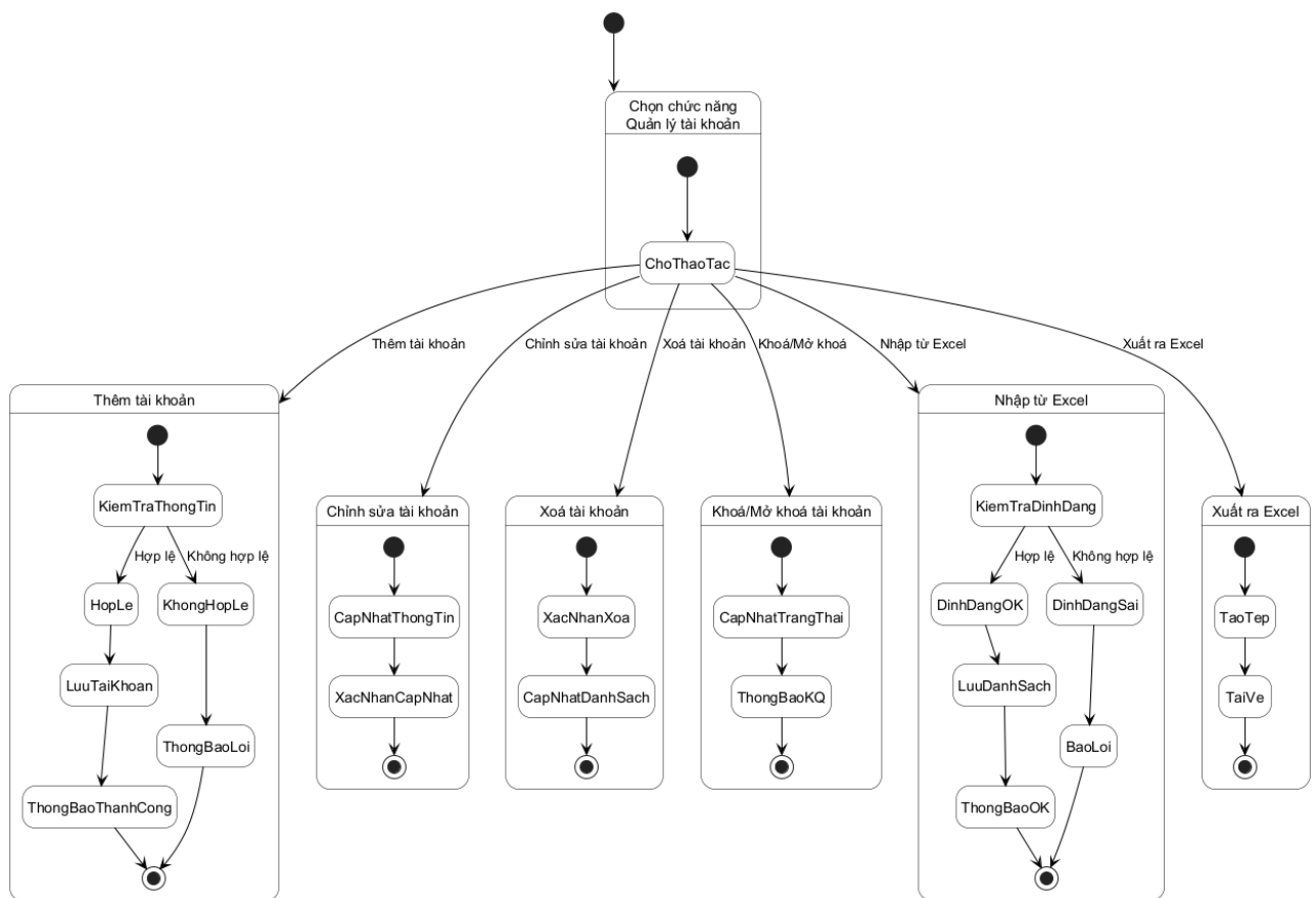
Hình 3.73: Sơ đồ trạng thái cho chức năng quản lý tài khoản
