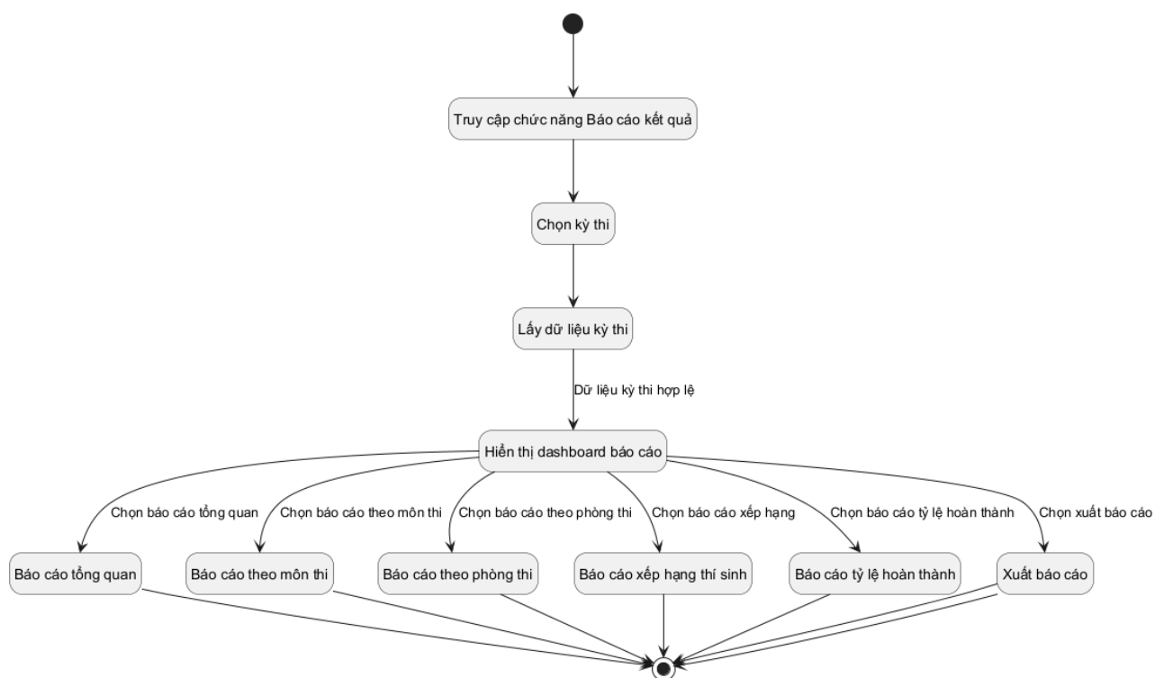
Hình 3.87: Sơ đồ trạng thái cho chức năng báo cáo thống kê
