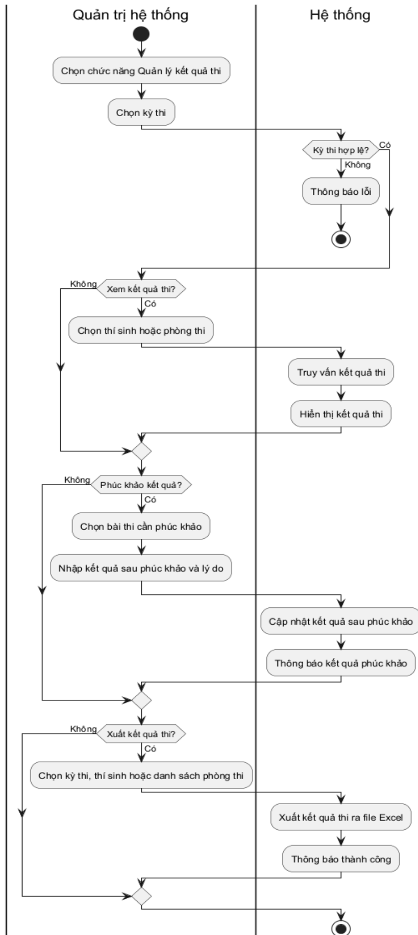
Hình 3.52: Sơ đồ hoạt động cho chức năng quản lý kết quả thi
