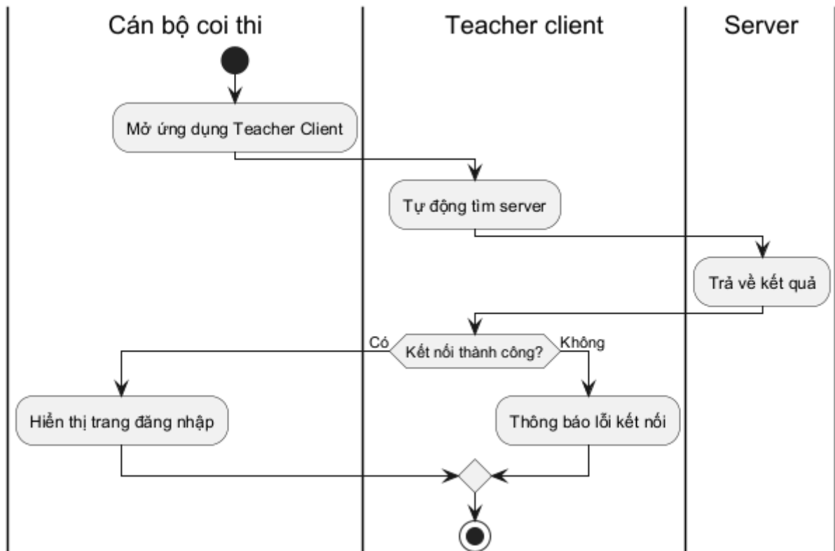
Hình 3.54: Sơ đồ hoạt động cho chức năng kết nối server
