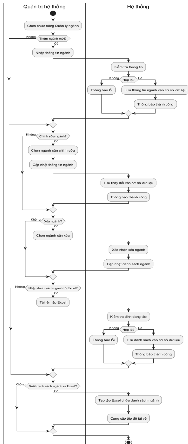
Hình 3.41: Sơ đồ hoạt động cho chức năng quản lý ngành
