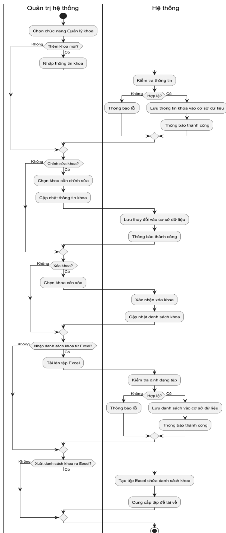
Hình 3.40: Sơ đồ hoạt động cho chức năng quản lý khoa
