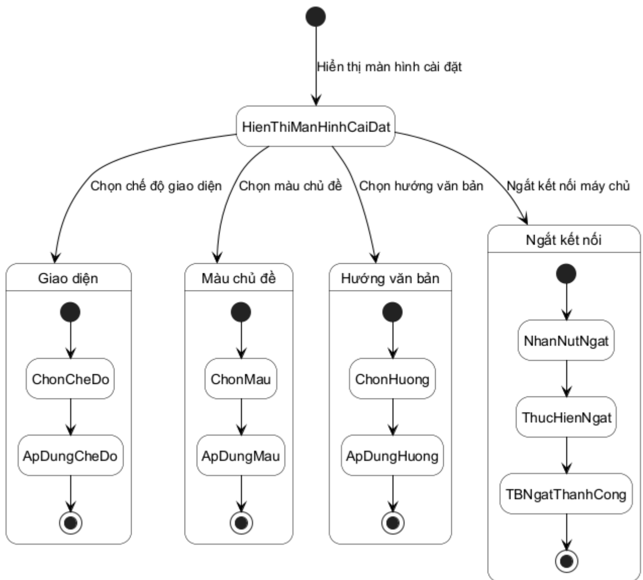
Hình 3.96: Sơ đồ trạng thái cho chức năng cài đặt ứng dụng teacher client
