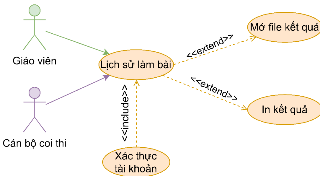
Hình 3.27: Phân rã use case lịch sử làm bài
