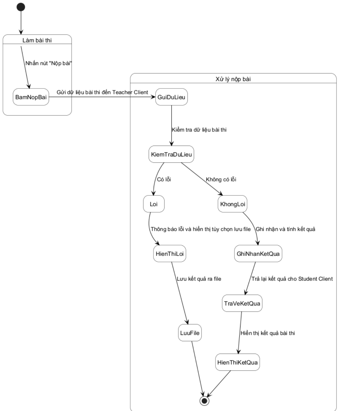
Hình 3.100: Sơ đồ trạng thái cho chức năng làm bài
