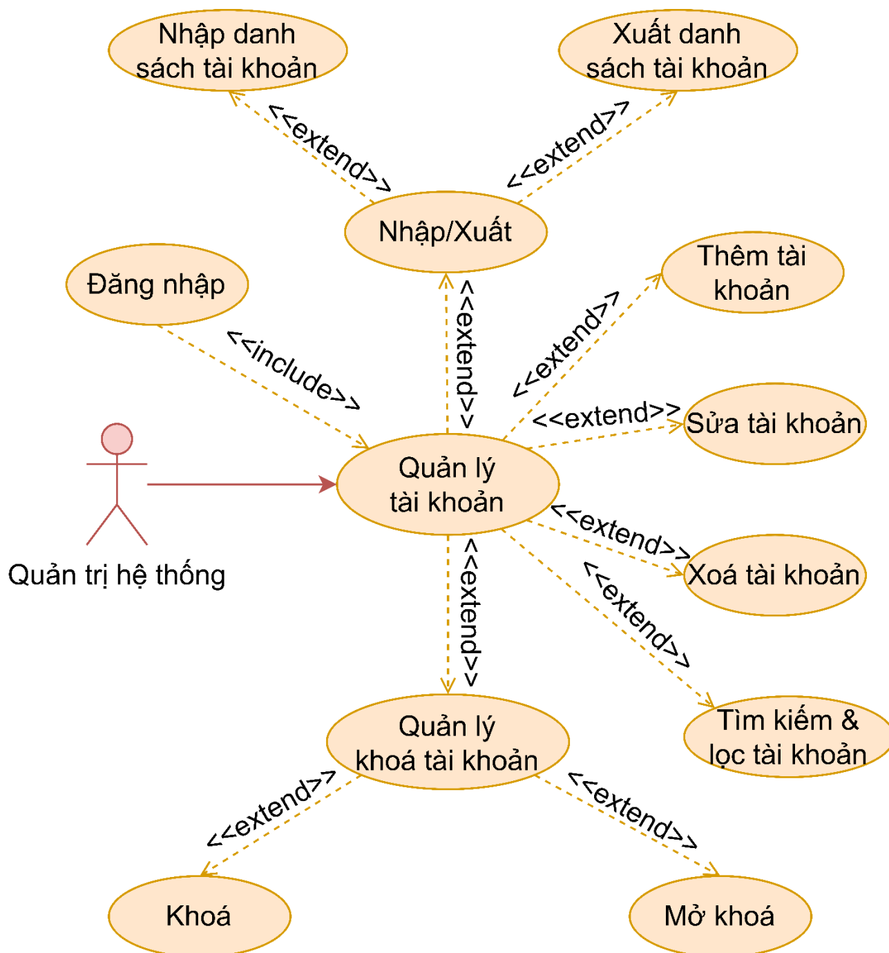
Hình 3.11: Phân rã use case Quản lý tài khoản
