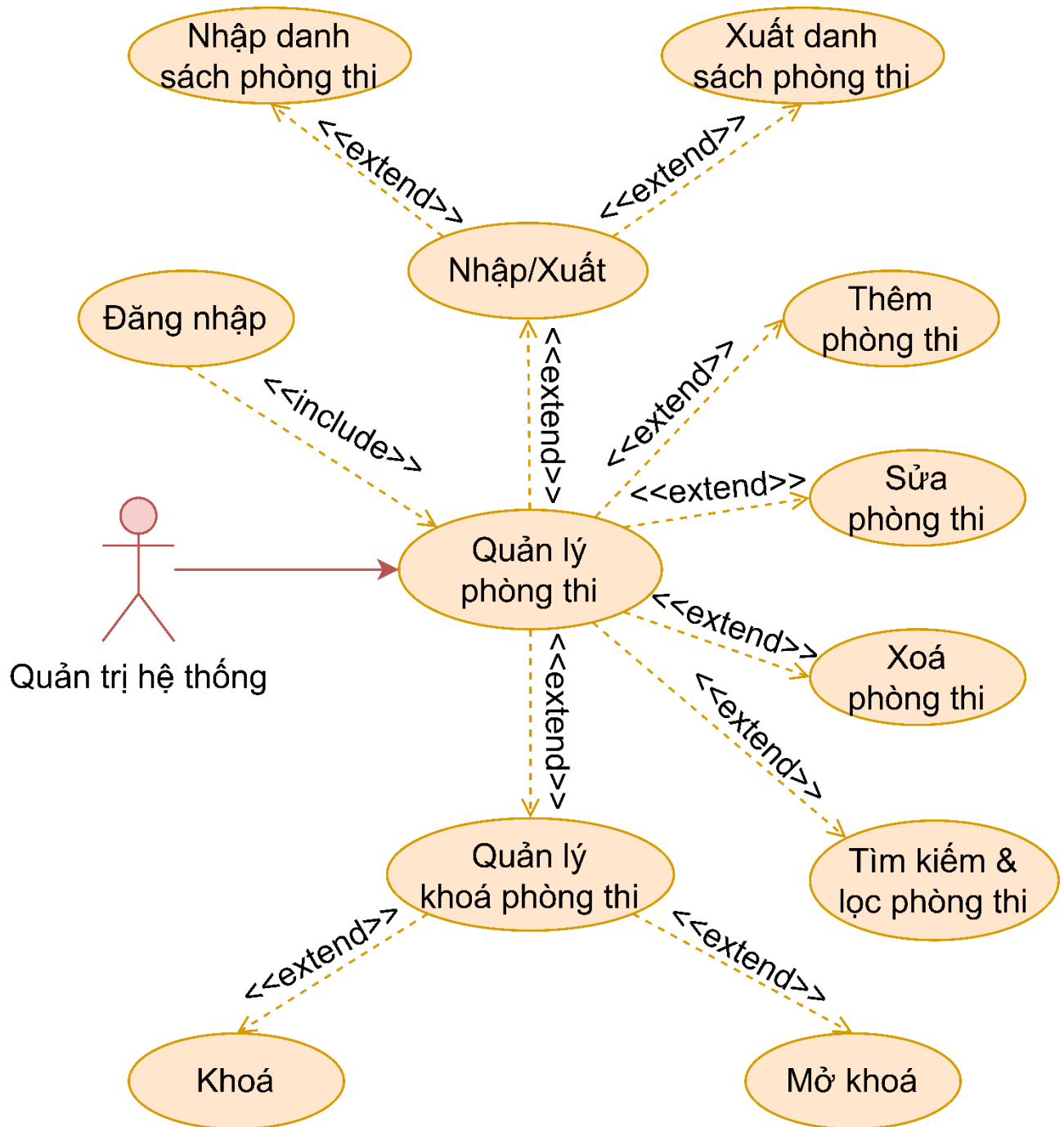
Hình 3.5: Phân rã use case Quản lý phòng thi
