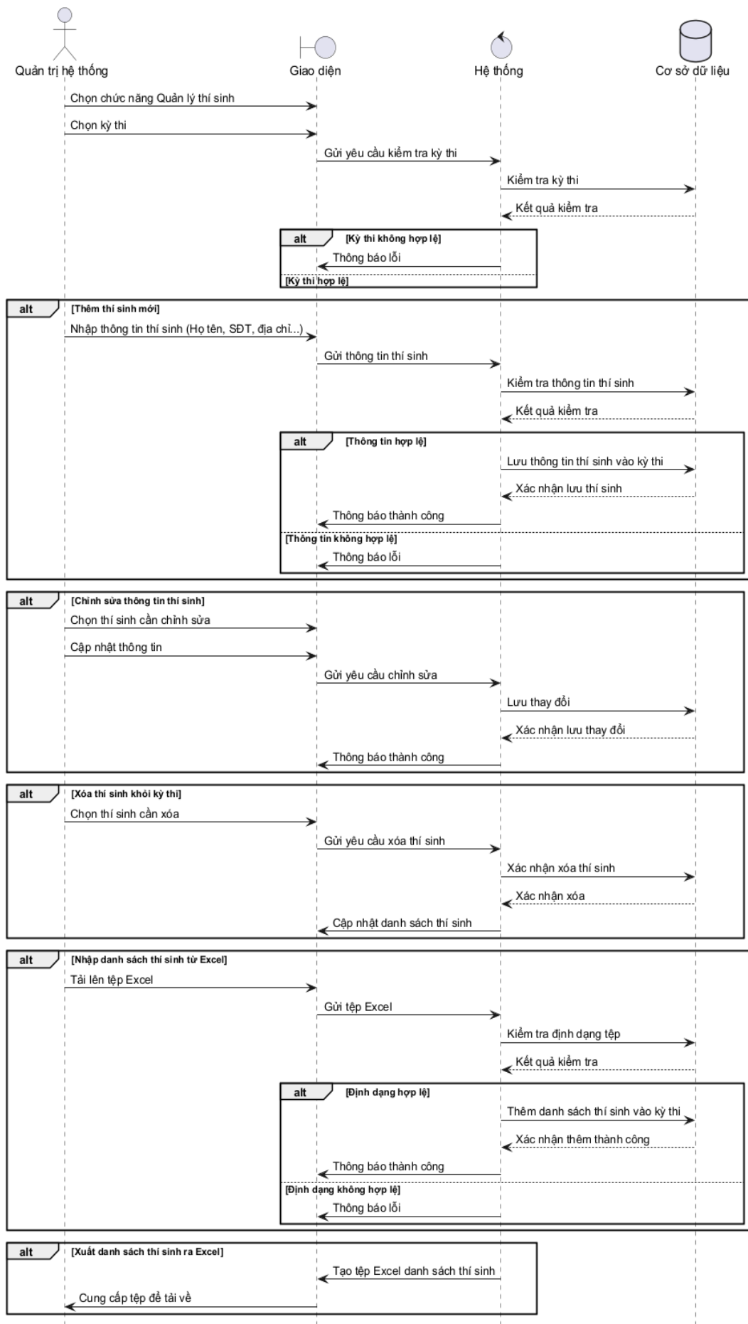
Hình 3.116: Sơ đồ tuần tự cho chức năng quản lý thí sinh
