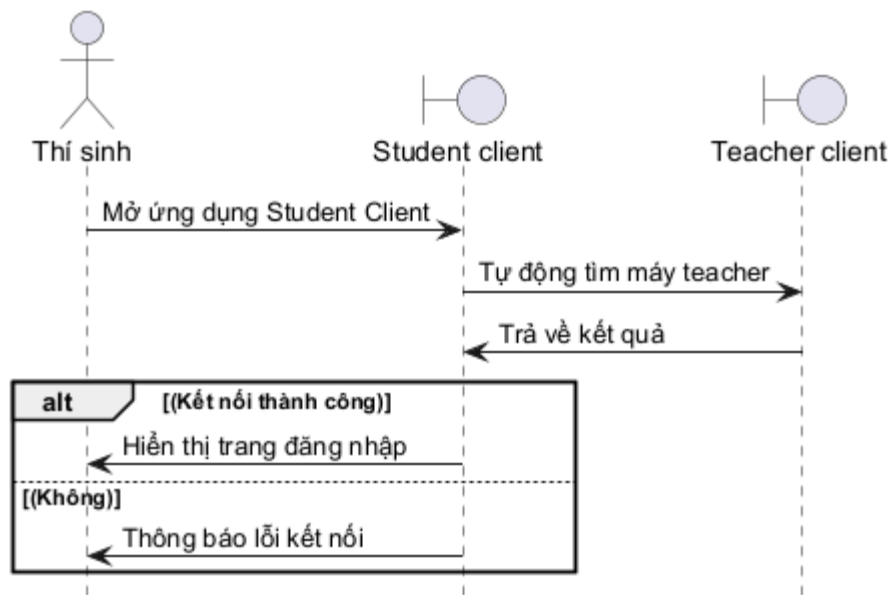
Hình 3.131: Sơ đồ tuần tự cho chức năng kết nối teacher client
