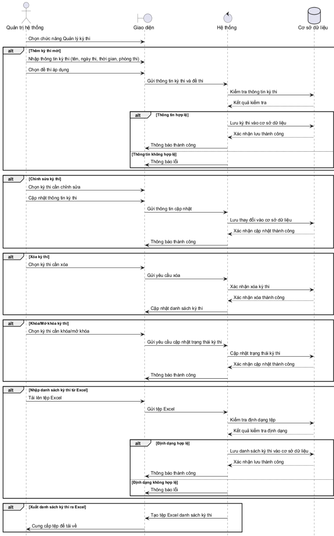
Hình 3.113: Sơ đồ tuần tự cho chức năng quản lý kỳ thi
