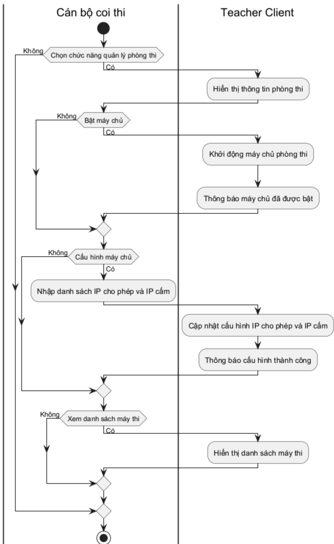
Hình 3.59: Sơ đồ hoạt động cho chức năng quản lý phòng thi
