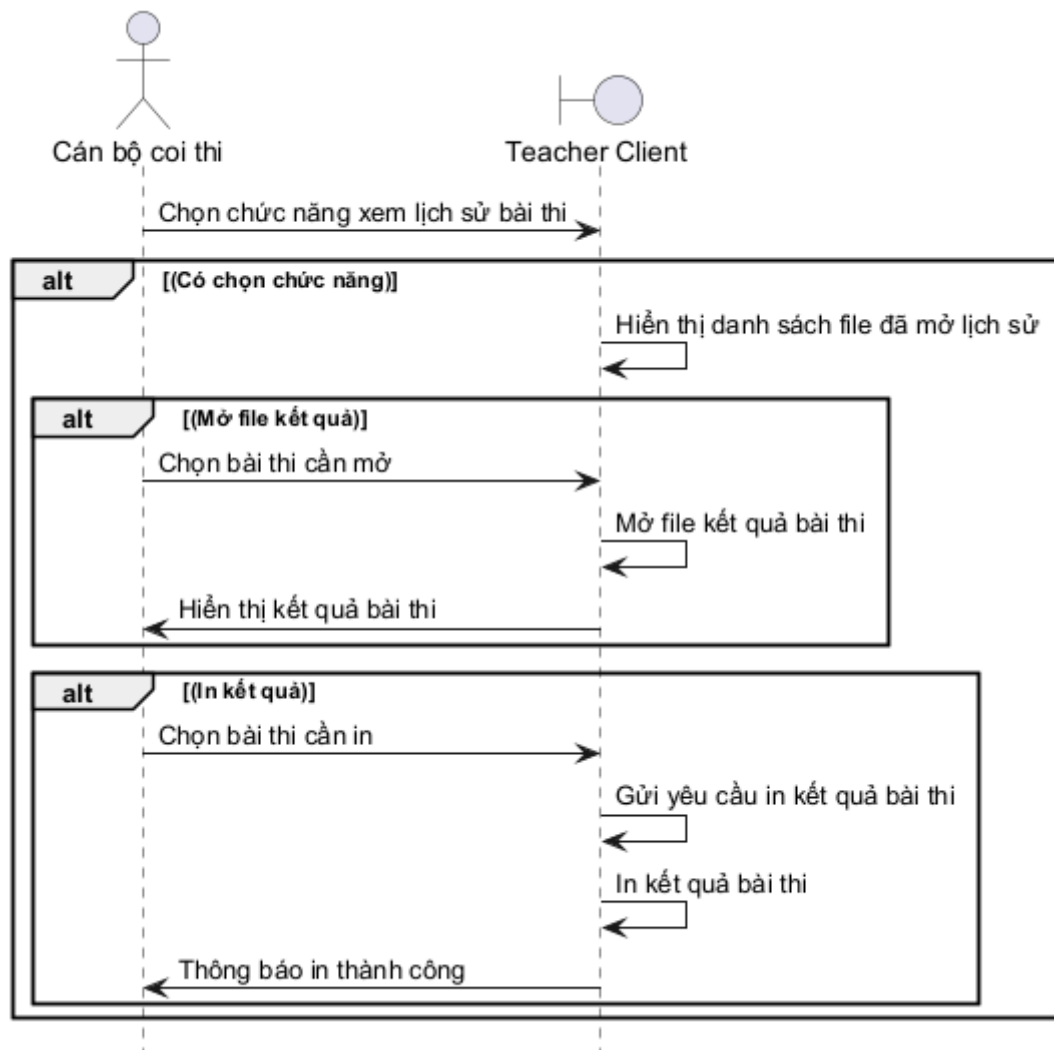
Hình 3.129: Sơ đồ tuần tự cho chức năng lịch sử bài thi
