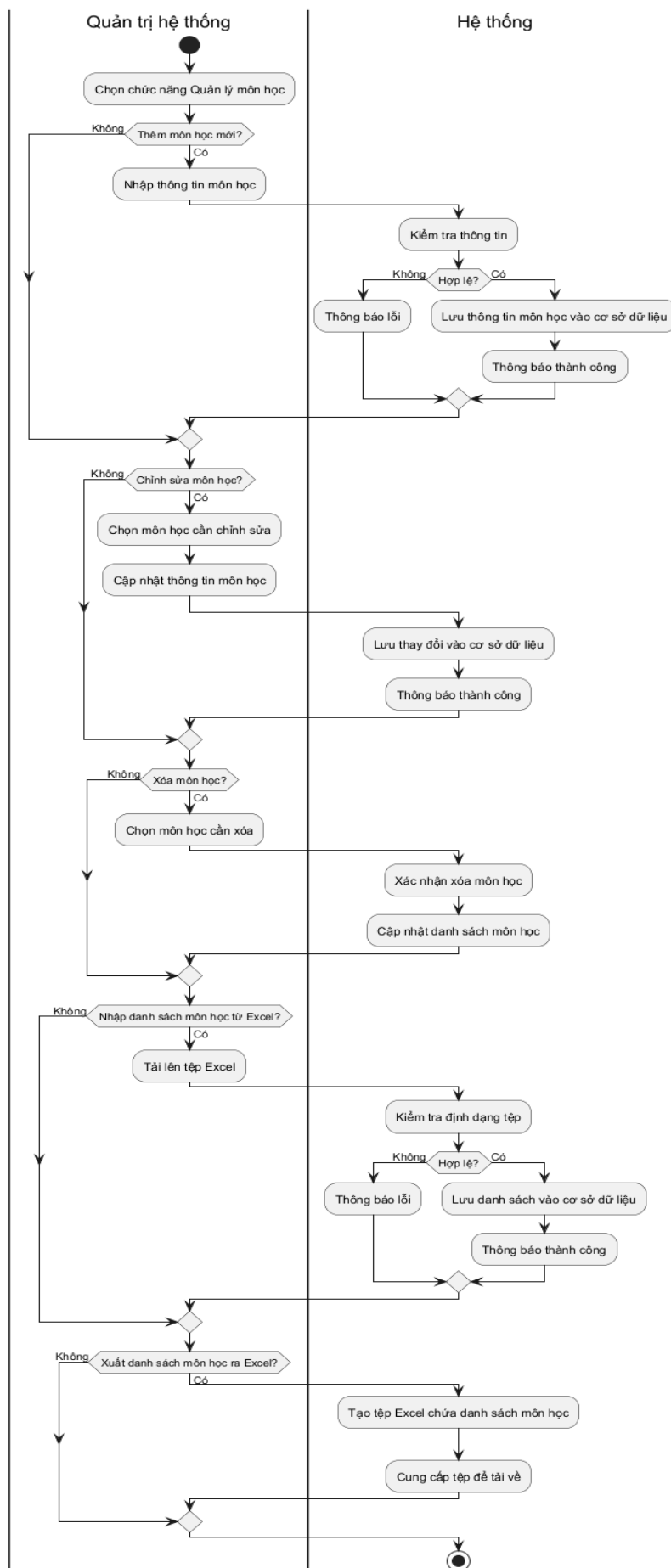
Hình 3.42: Sơ đồ hoạt động cho chức năng quản lý môn học
