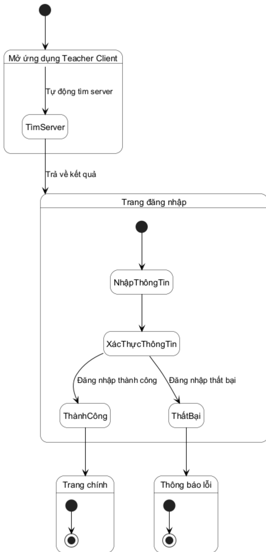
Hình 3.88: Sơ đồ trạng thái cho chức năng kết nối server
