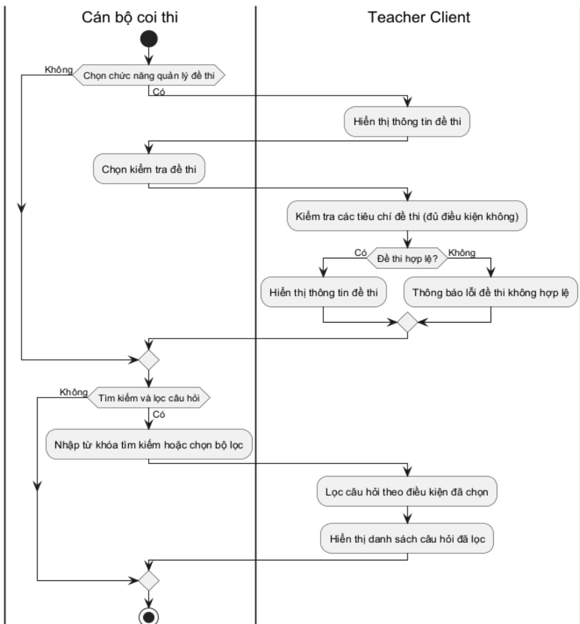
Hình 3.57: Sơ đồ hoạt động cho chức năng quản lý đề thi
