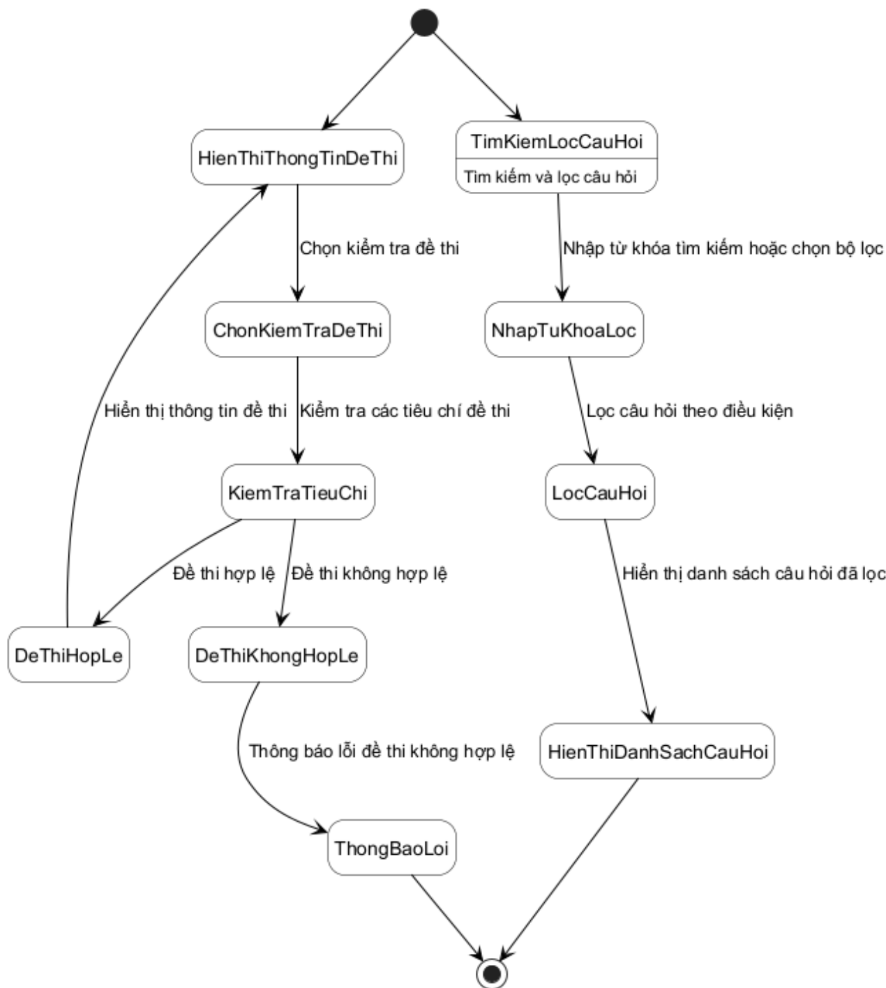
Hình 3.91: Sơ đồ trạng thái cho chức năng quản lý đề thi
