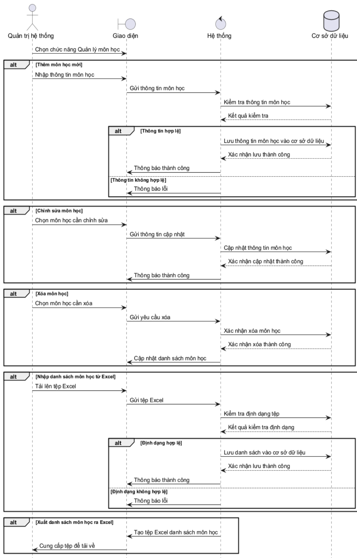
Hình 3.110: Sơ đồ tuần tự cho chức năng quản lý môn học
