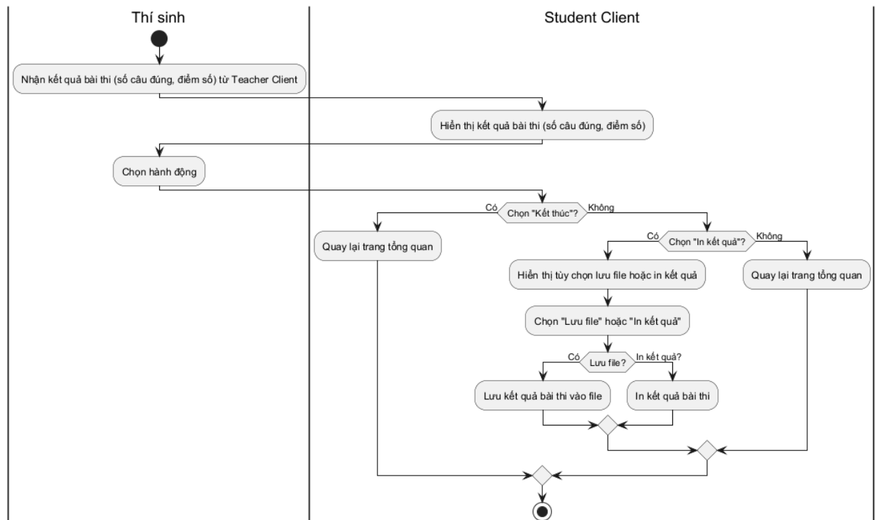
Hình 3.67: Sơ đồ hoạt động cho chức năng kết quả
