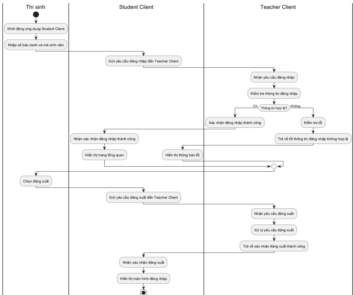
Hình 3.64: Sơ đồ hoạt động cho chức năng xác thực thí sinh
