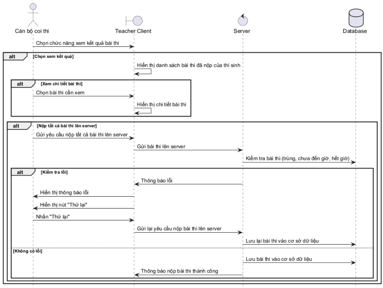
Hình 3.128: Sơ đồ tuần tự cho chức năng kết quả bài thi
