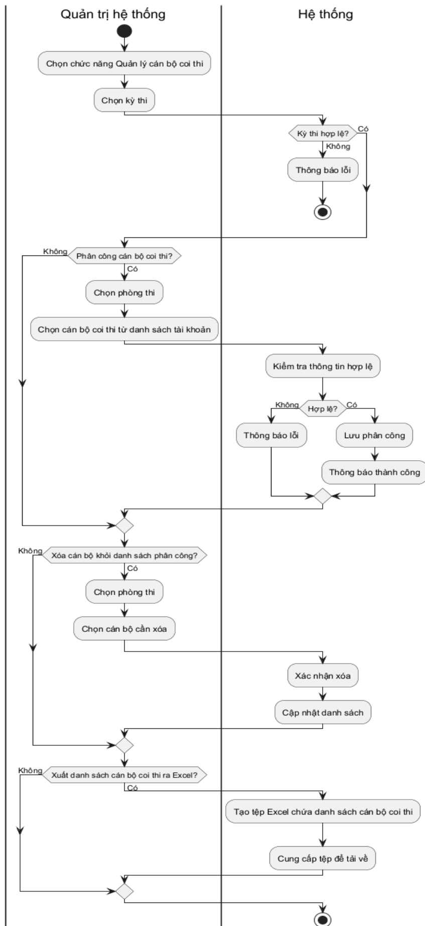
Hình 3.49: Sơ đồ hoạt động cho chức năng quản lý cán bộ coi thi
