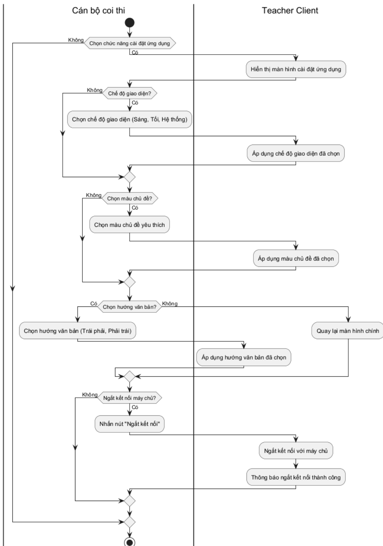
Hình 3.62: Sơ đồ hoạt động cho chức năng cài đặt ứng dụng teacher client
