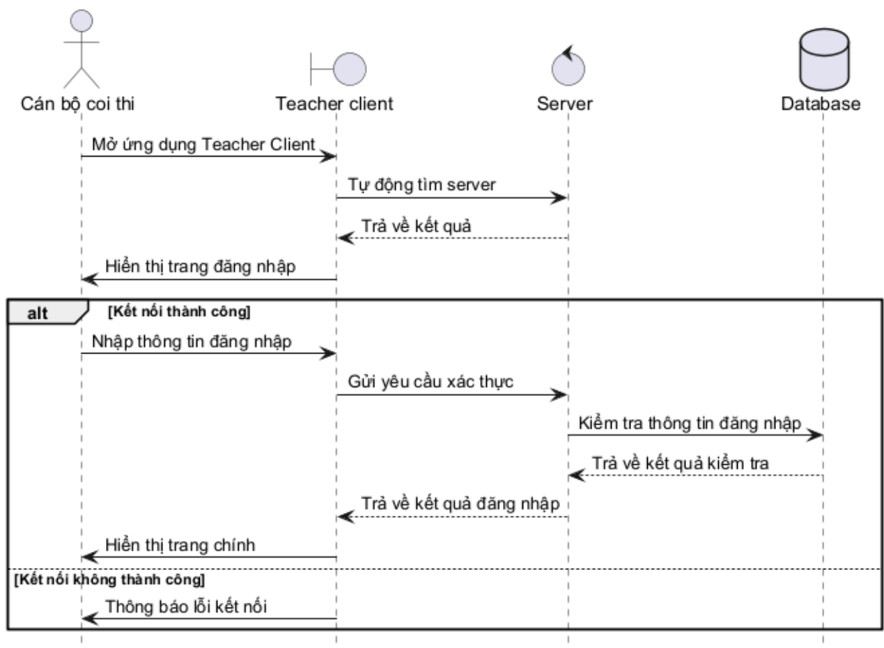
Hình 3.122: Sơ đồ tuần tự cho chức năng kết nối server
