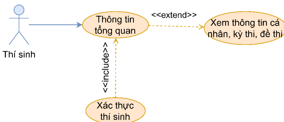
Hình 3.32: Phân rã use case thông tin tổng quan
