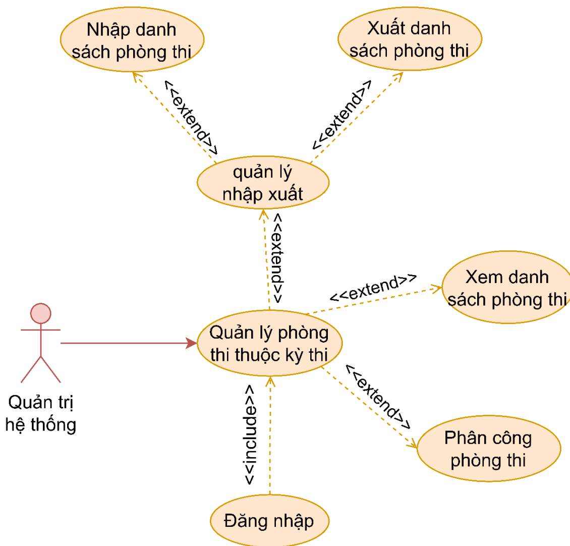
Hình 3.17: Phân rã use case quản lý phòng thi thuộc kỳ thi
