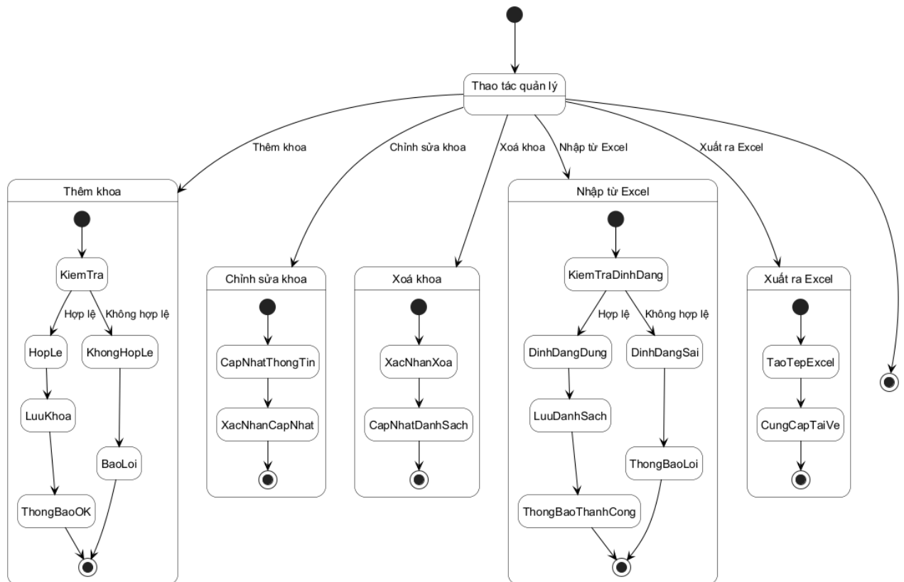
Hình 3.74: Sơ đồ trạng thái cho chức năng quản lý khóa
