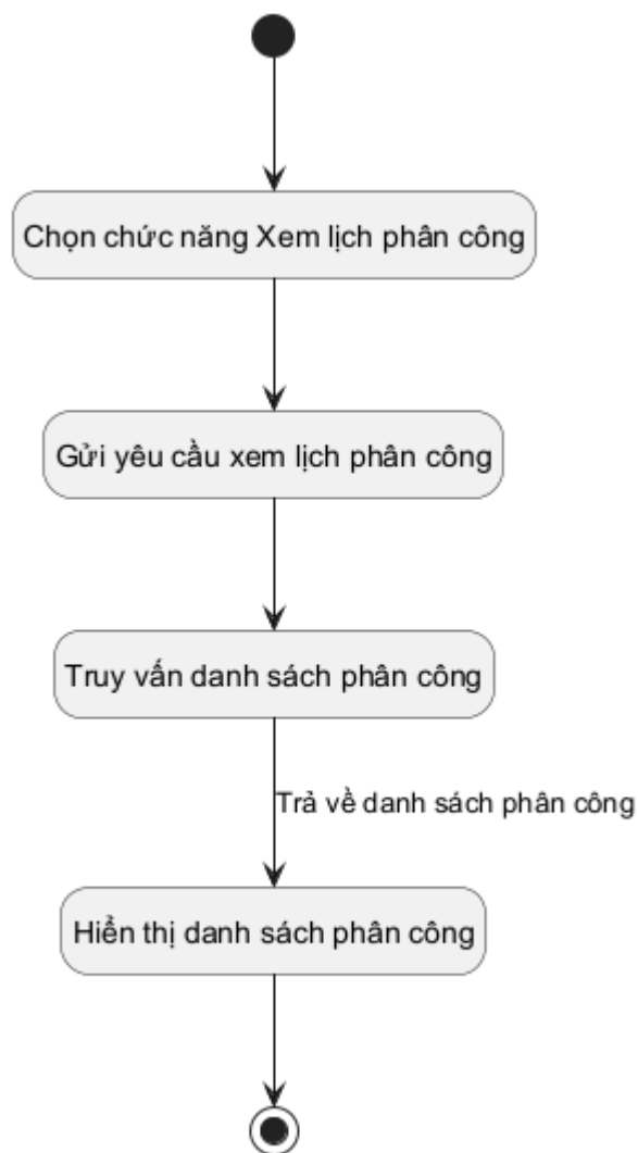
Hình 3.70: Sơ đồ trạng thái cho chức năng xem lịch phân công
