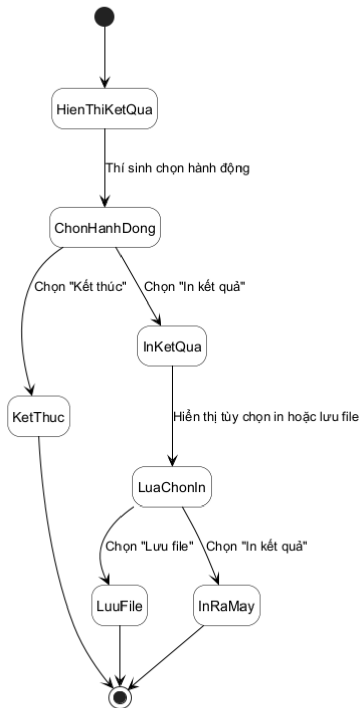
Hình 3.101: Sơ đồ trạng thái cho chức năng kết quả
