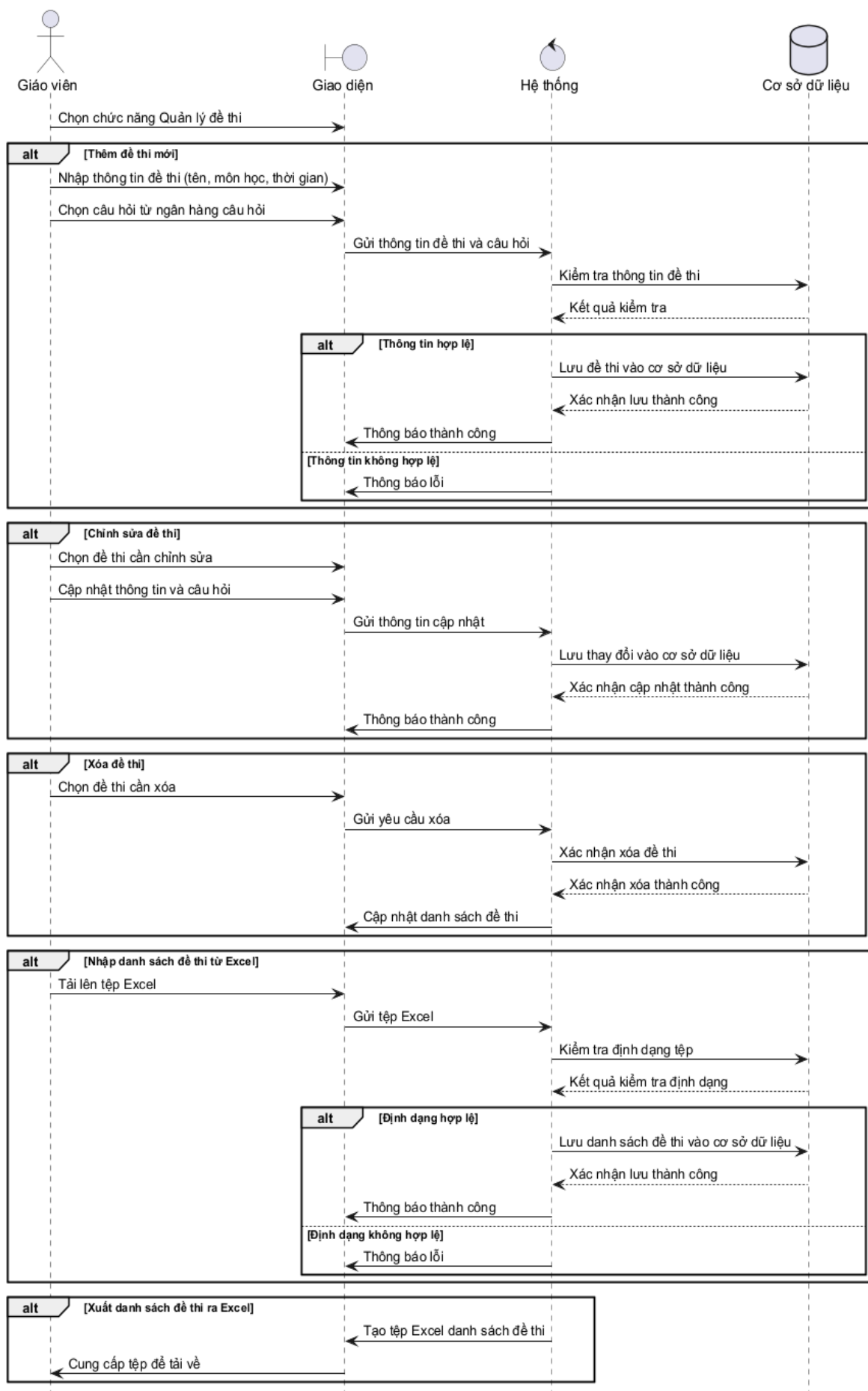
Hình 3.112: Sơ đồ tuần tự cho chức năng quản lý đề thi
