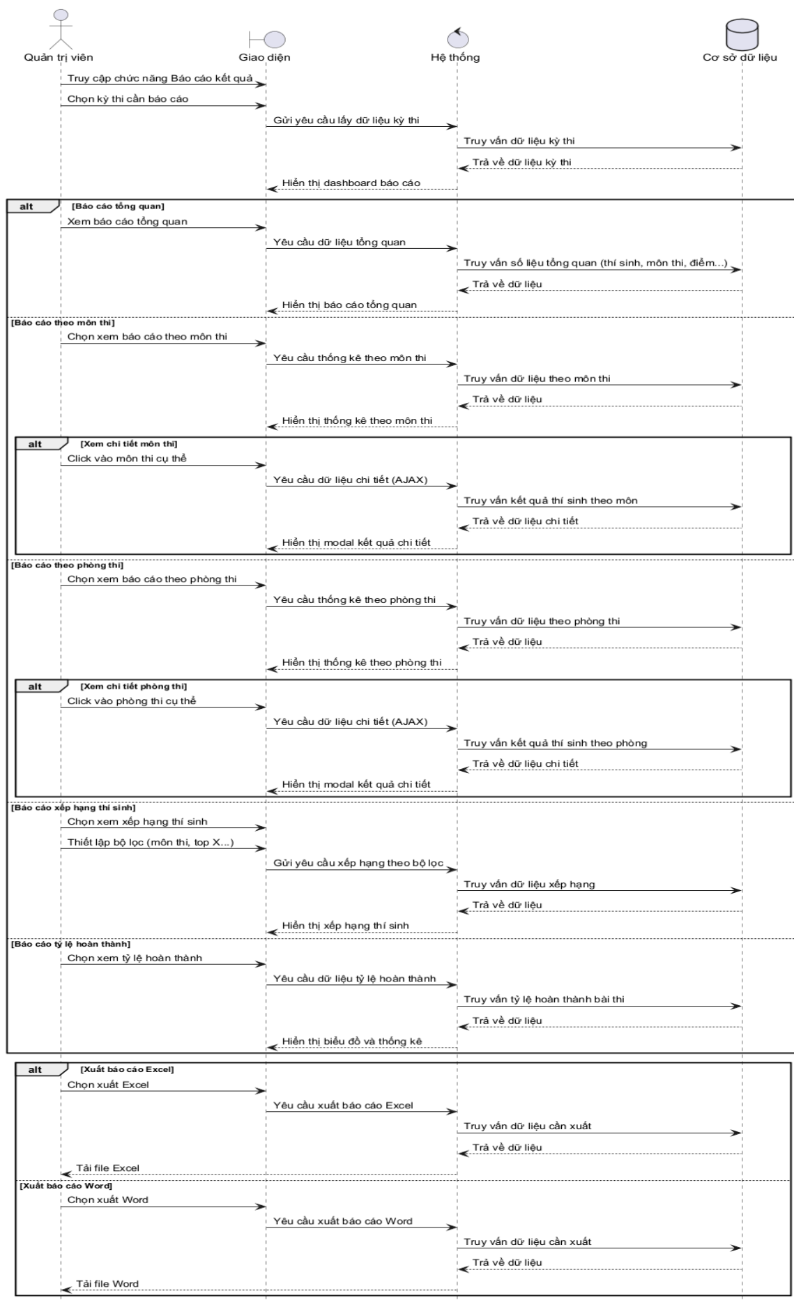
Hình 3.121: Sơ đồ tuần tự cho chức năng báo cáo thống kê
