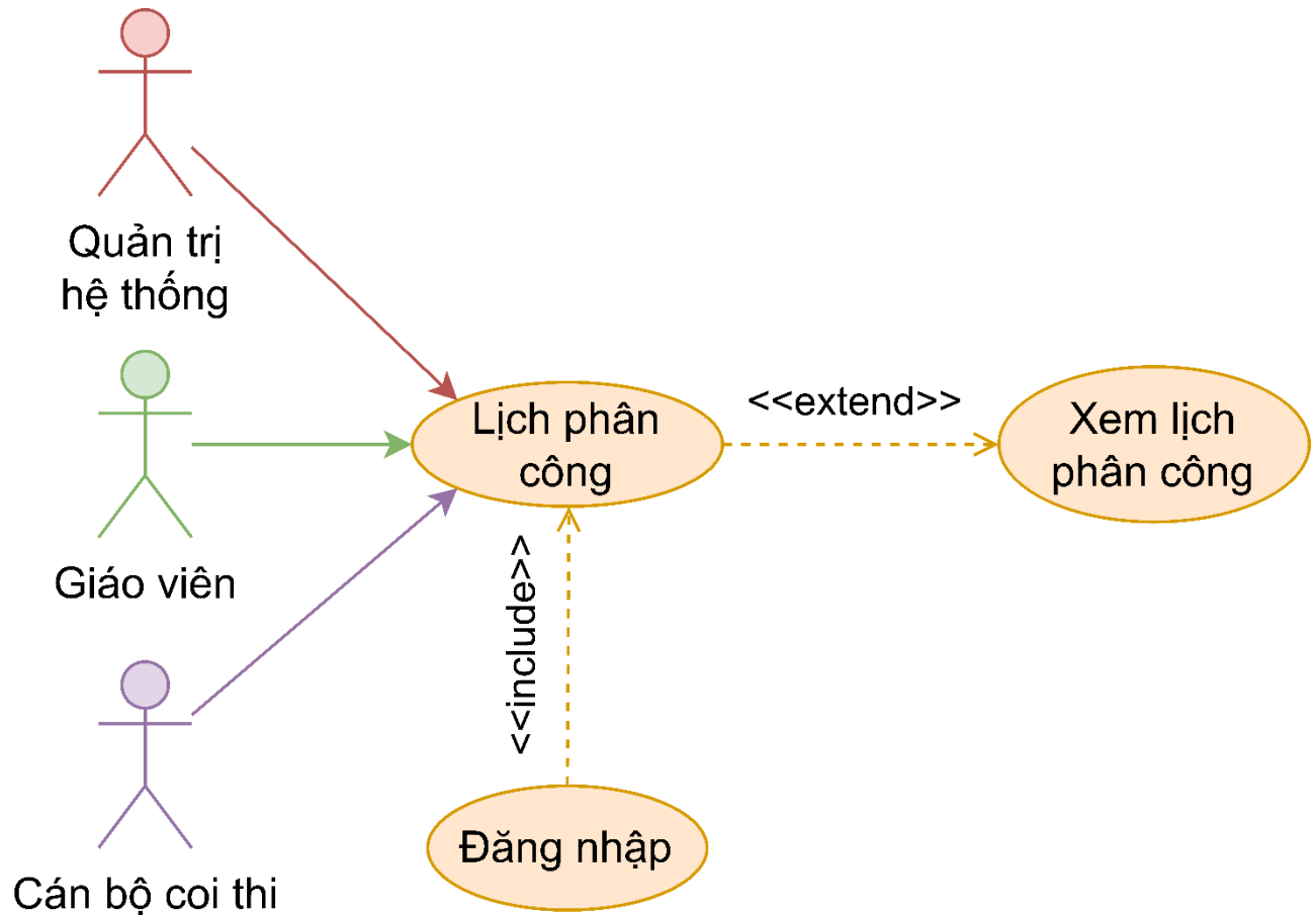
Hình 3.3: Phân rã use case Lịch phân công
