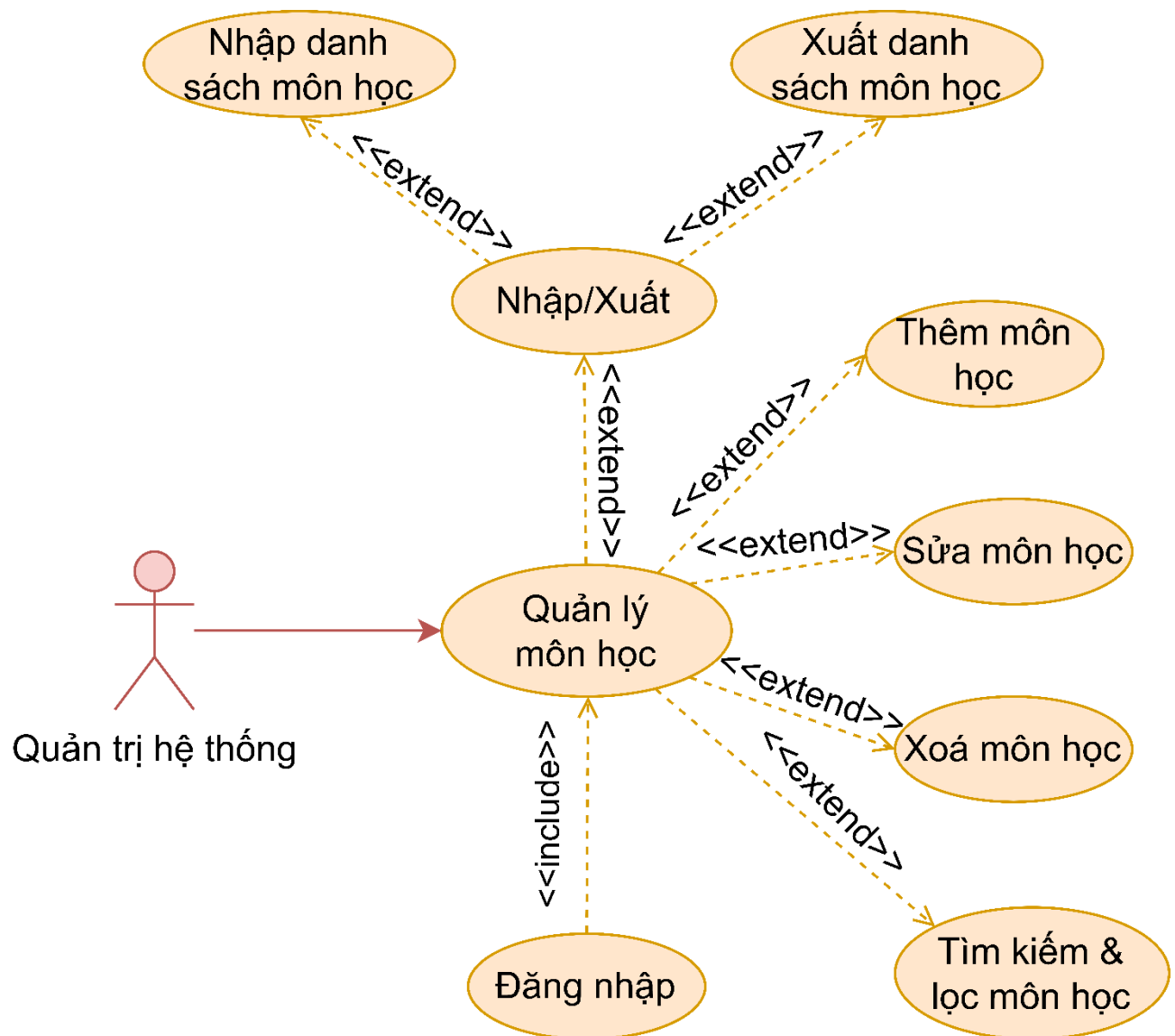
Hình 3.8: Phân rã use case Quản lý môn học
