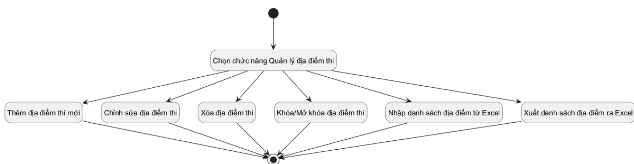
Hình 3.71: Sơ đồ trạng thái cho chức năng quản lý địa điểm
