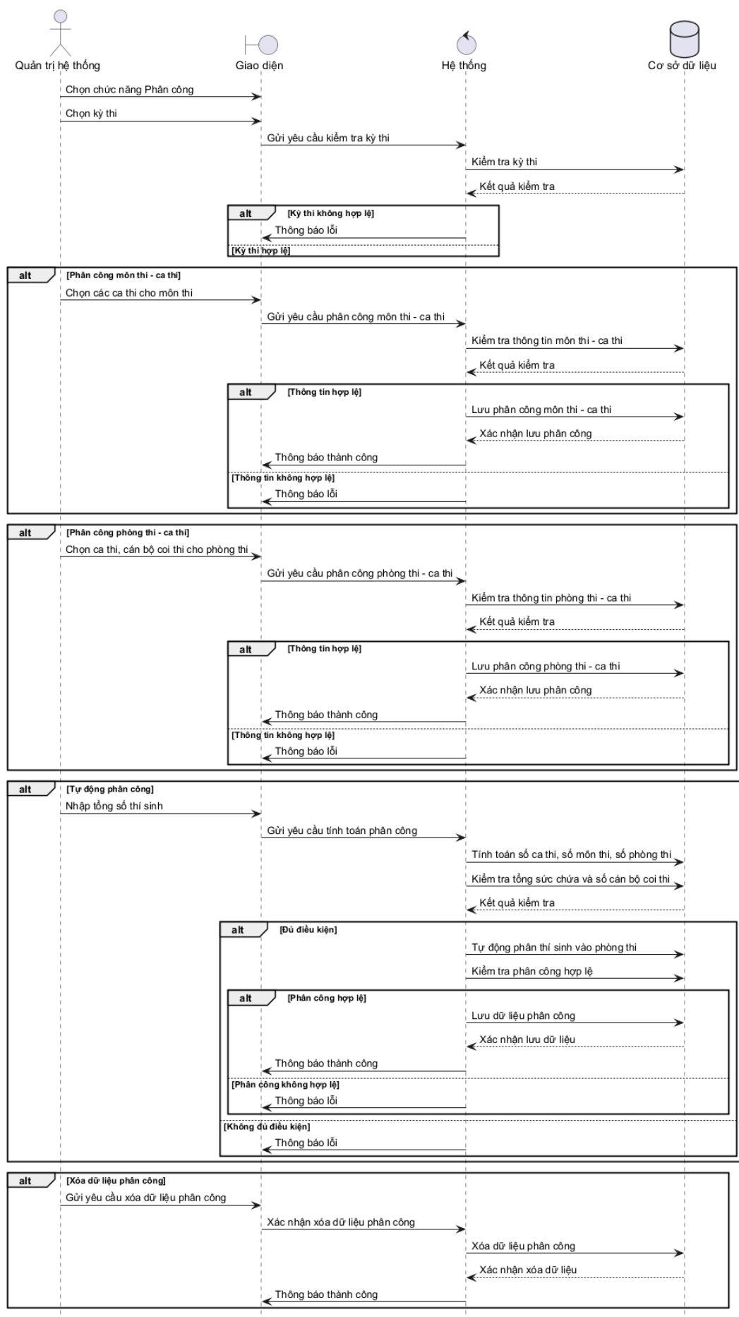
Hình 3.119: Sơ đồ tuần tự cho chức năng phân công
