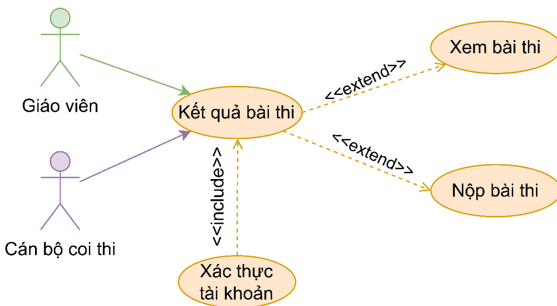
Hình 3.26: Phân rã use case Kết quả bài thi
