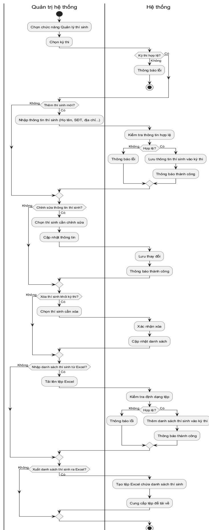
Hình 3.48: Sơ đồ hoạt động cho chức năng quản lý thí sinh
