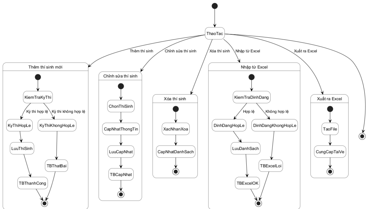
Hình 3.82: Sơ đồ trạng thái cho chức năng quản lý thí sinh
