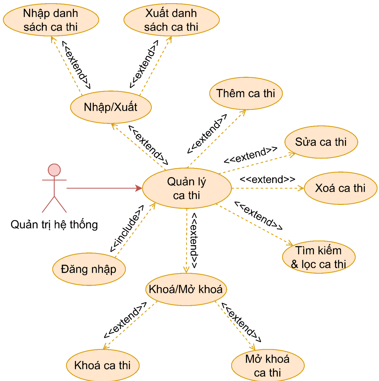
Hình 3.13: Phân rã use case Quản ca thi
