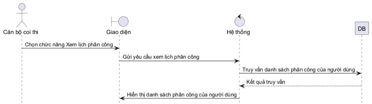
Hình 3.104: Sơ đồ tuần tự cho chức năng xem lịch phân công
