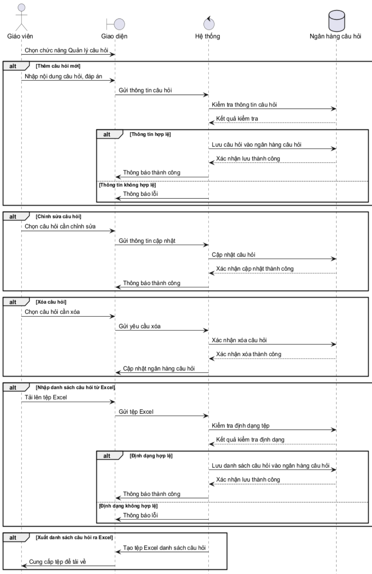
Hình 3.111: Sơ đồ tuần tự cho chức năng quản lý câu hỏi
