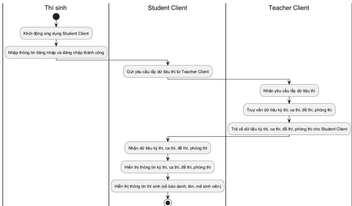
Hình 3.65: Sơ đồ hoạt động cho chức năng tổng quan bài thi
