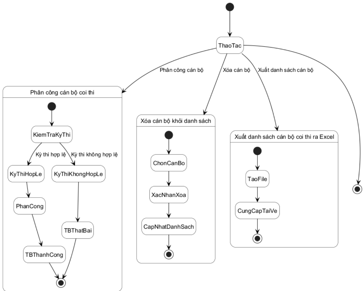
Hình 3.83: Sơ đồ trạng thái cho chức năng quản lý cán bộ coi thi
