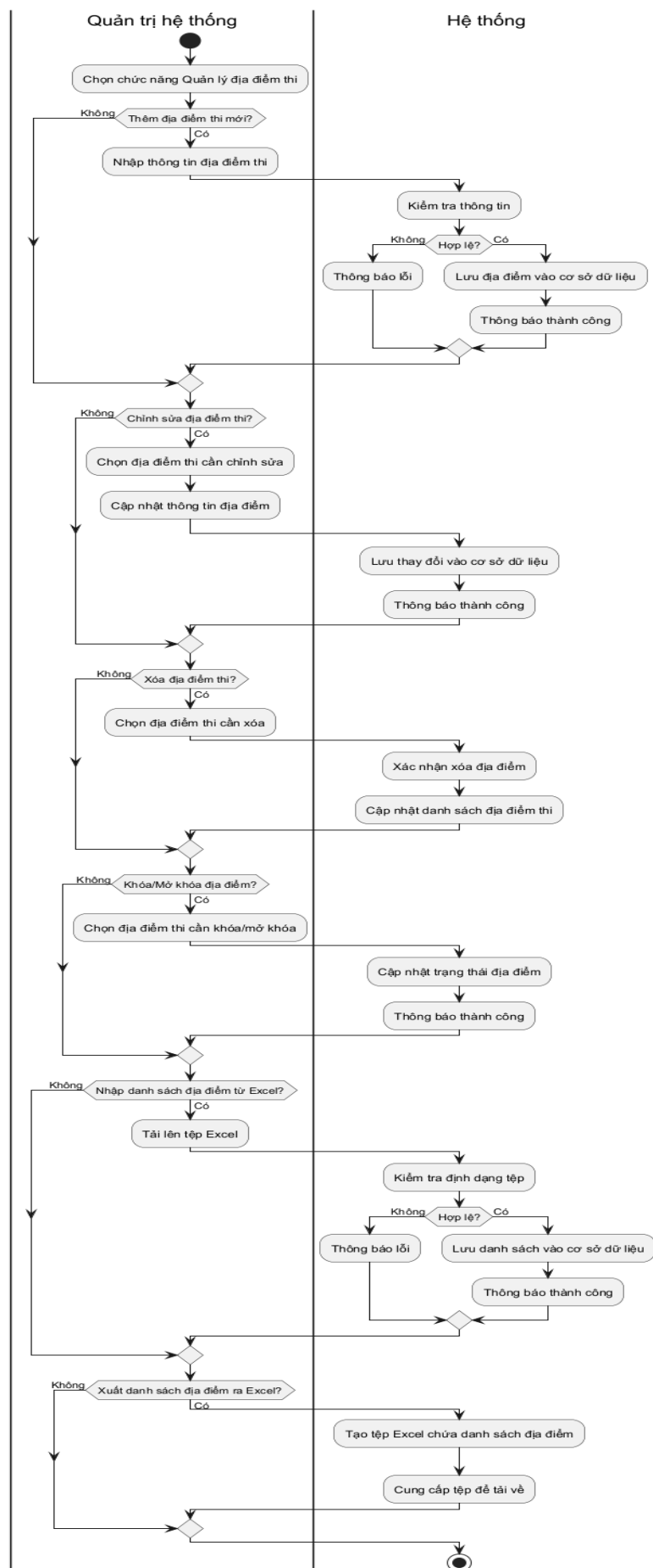
Hình 3.37: Sơ đồ hoạt động cho chức năng quản lý địa điểm
