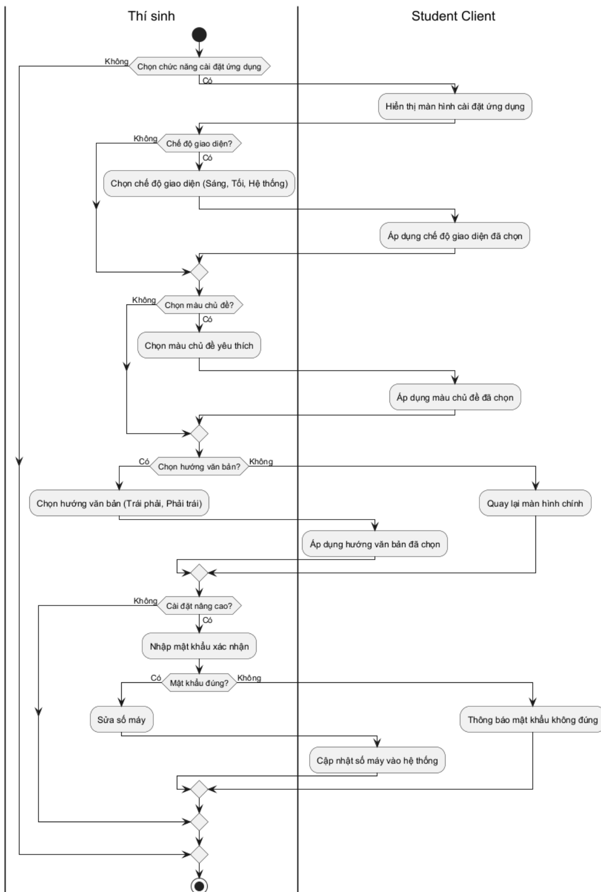
Hình 3.68: Sơ đồ hoạt động cho chức năng cài đặt ứng dụng student client
