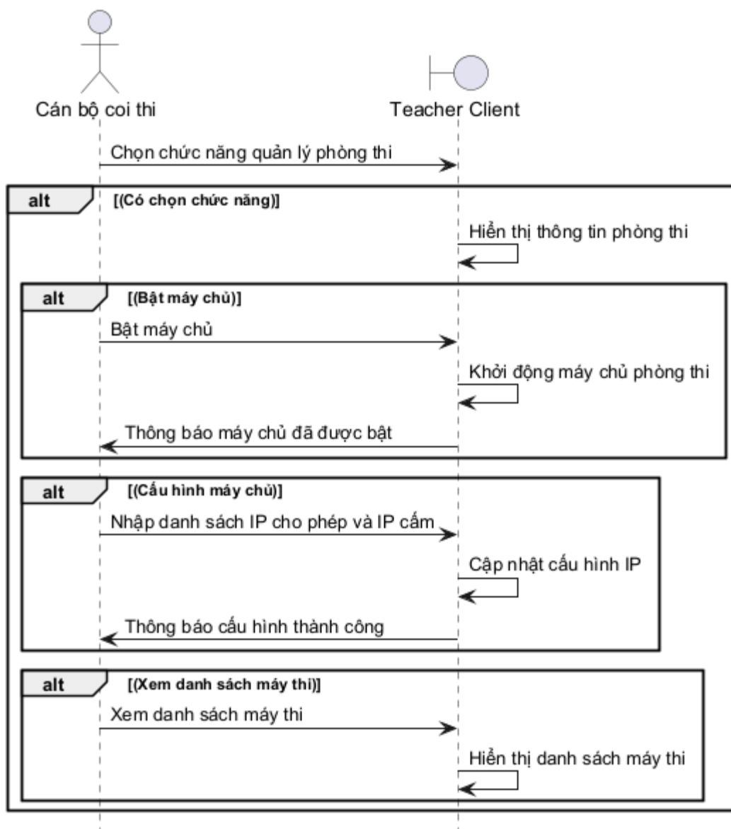
Hình 3.127: Sơ đồ tuần tự cho chức năng quản lý phòng thi
