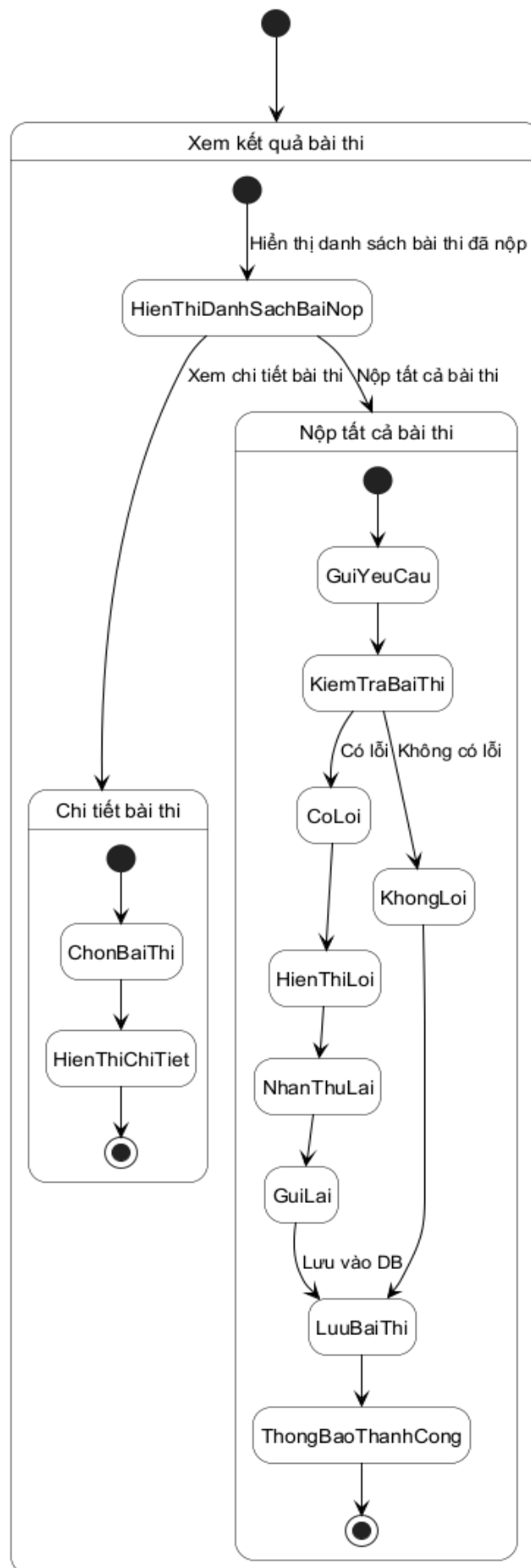
Hình 3.94: Sơ đồ trạng thái cho chức năng kết quả bài thi
