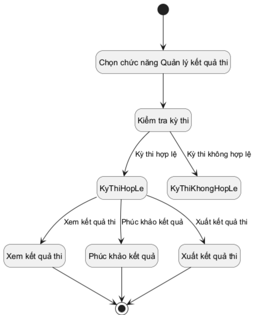
Hình 3.86: Sơ đồ trạng thái cho chức năng quản lý kết quả thi
