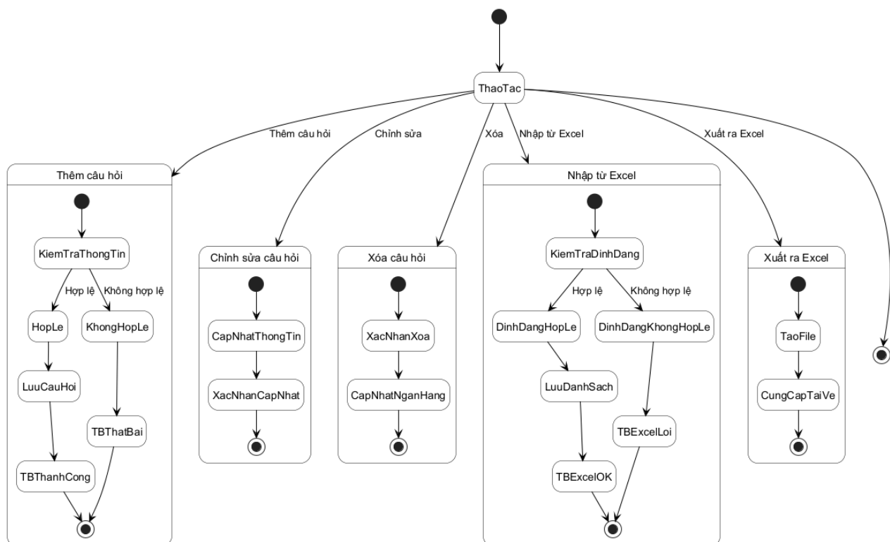
Hình 3.77: Sơ đồ trạng thái cho chức năng quản lý câu hỏi
