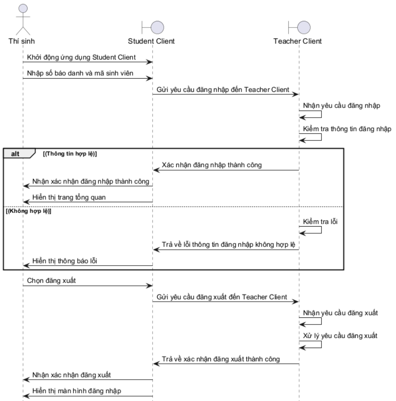
Hình 3.132: Sơ đồ tuần tự cho chức năng xác thực thí sinh
