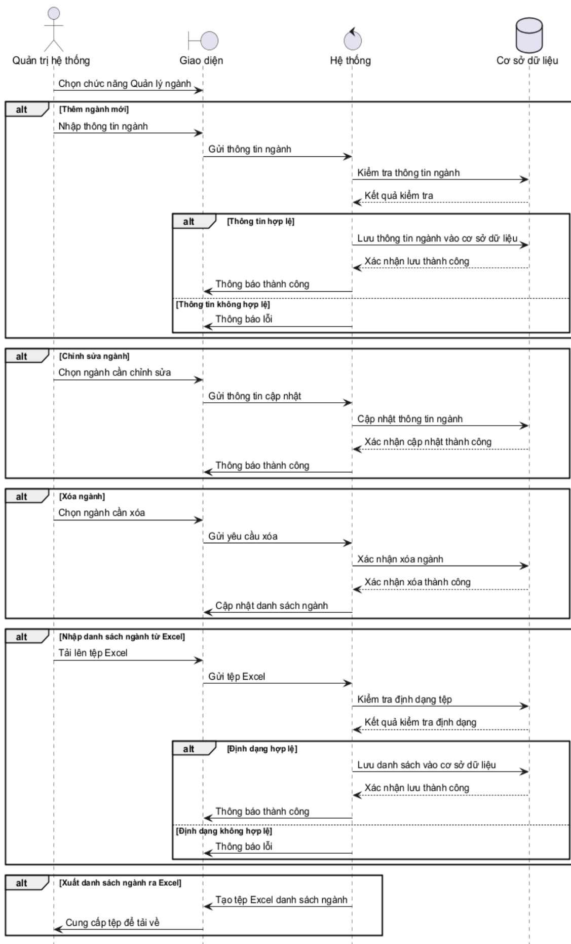
Hình 3.109: Sơ đồ tuần tự cho chức năng quản lý ngành
